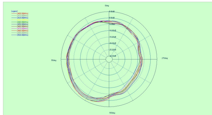
RX1: \Phi=90^\circ
