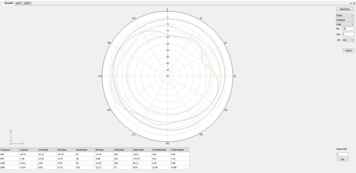
GSM 850/WCDMA B5/B20 LTE B5 NR n5/n20 Theta=90deg
