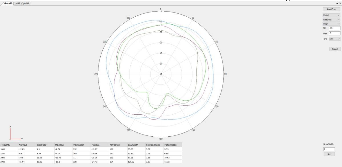
WCDMA B1/B4/LTE B1/B4/B7/B38/B41 NR n1/n7/n38/n41 Theta=90deg
