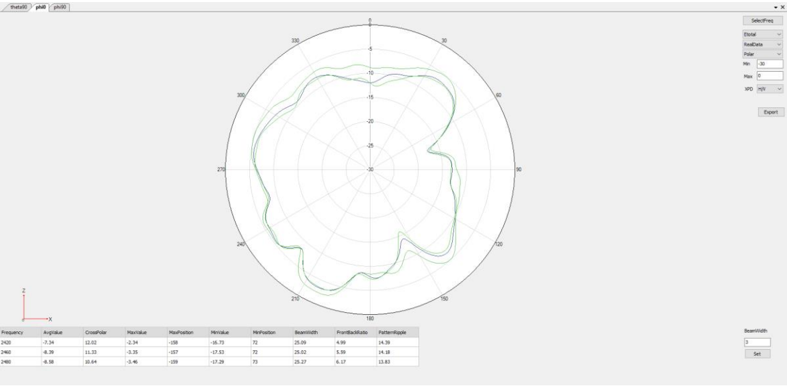
WIFI2.4 Phi=0deg
