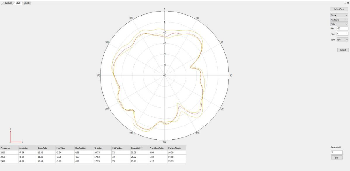
GPS(L1)/WIFI2.4 Phi=0deg
