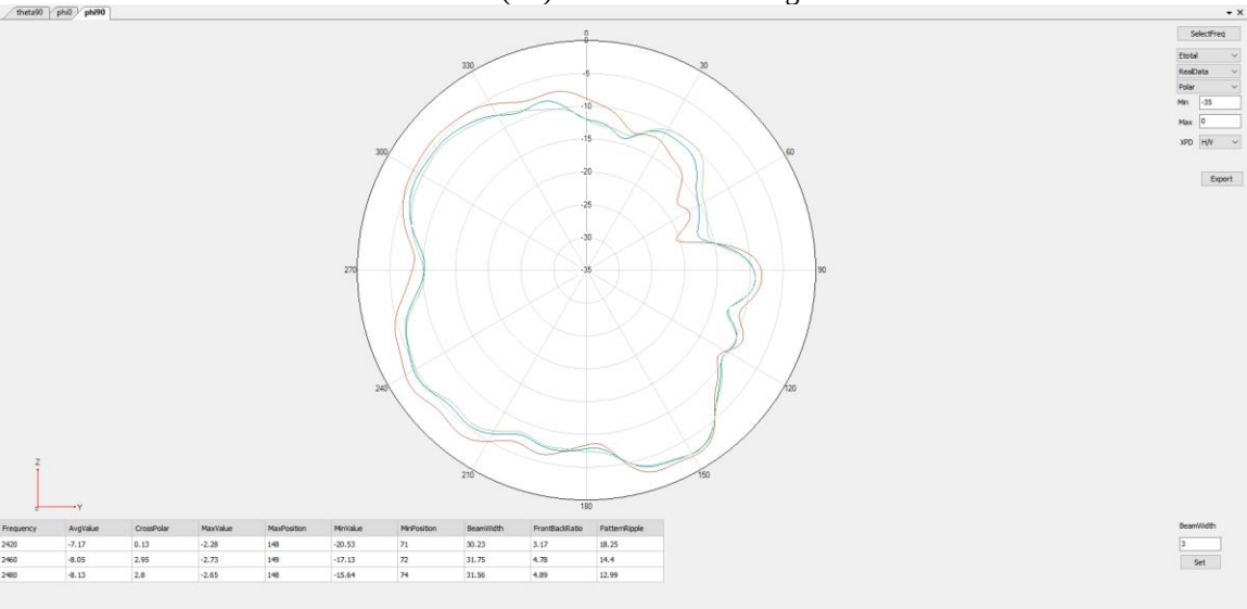
GPS(L1)/WIFI2.4Phi=90deg
