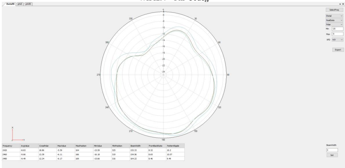
WIFI2.4 Theta=90deg
