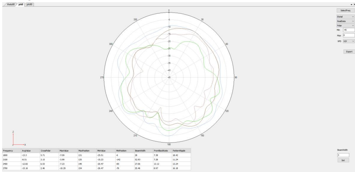
WCDMA B1/B4/LTE B1/B4/B7/B38/B41NR n1/n7/n38/n41 Phi=0deg
