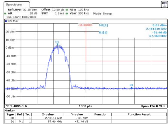
802.11b_2462MHz_Chain 0
