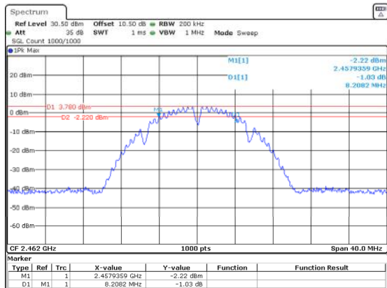
802.11b_2462MHz_Chain 0
