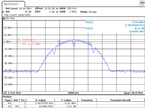
802.11b_2412MHz_Chain 0
