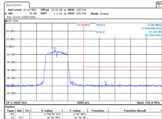
802.11n20_2462MHz_Chain 0
