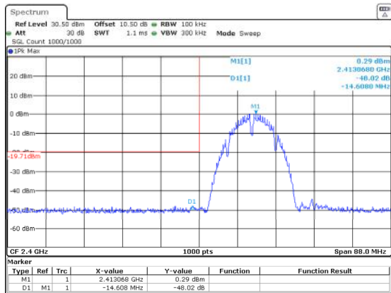
802.11b_2412MHz_Chain 1
