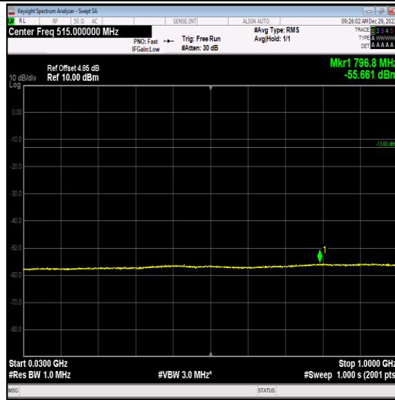
Band4-1312-5-30~1000MHz-PASS
