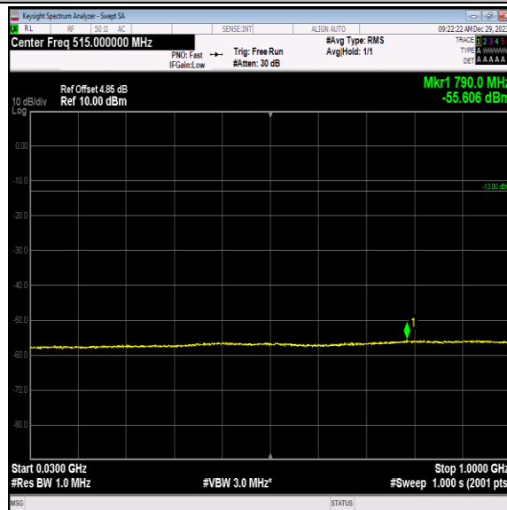
Band4-1312-4-30~1000MHz-PASS
