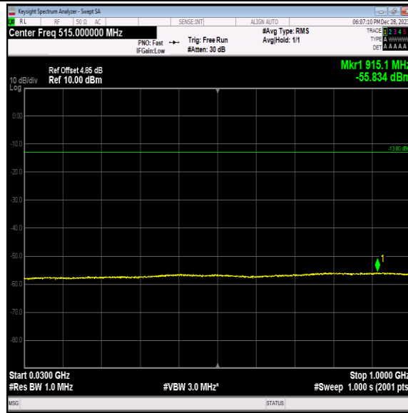
Band2-9538-5-30~1000MHz-PASS
