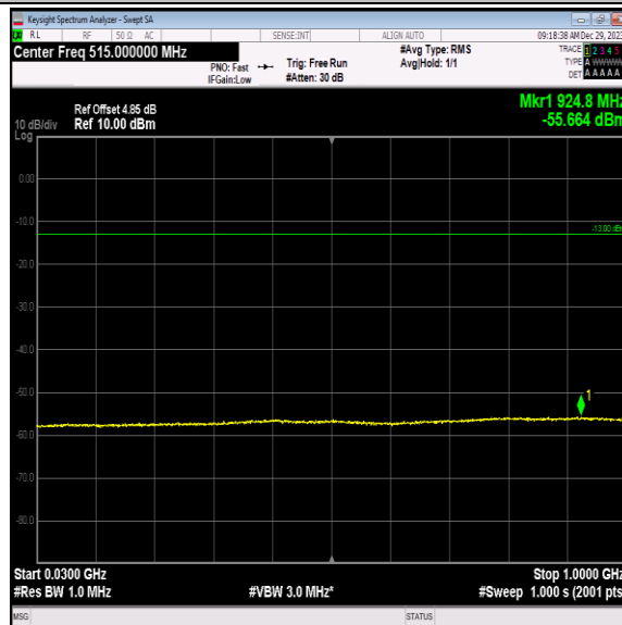
Band4-1312-3-30~1000MHz-PASS
