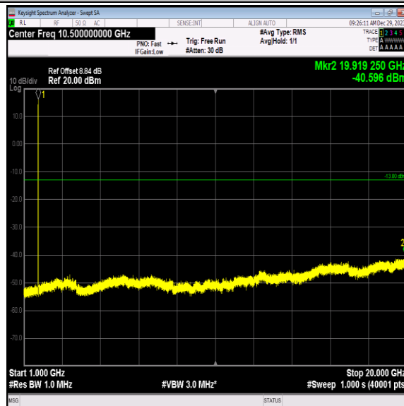
Band4-1312-5-1000~20000MHz-PASS
