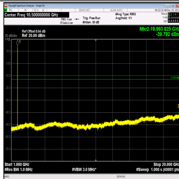
Band4-1312-4-1000~20000MHz-PASS
