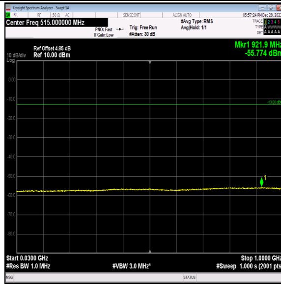
Band2-9538-2-30~1000MHz-PASS
