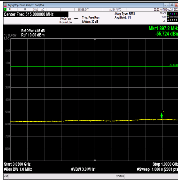
Band2-9538-1-30~1000MHz-PASS
