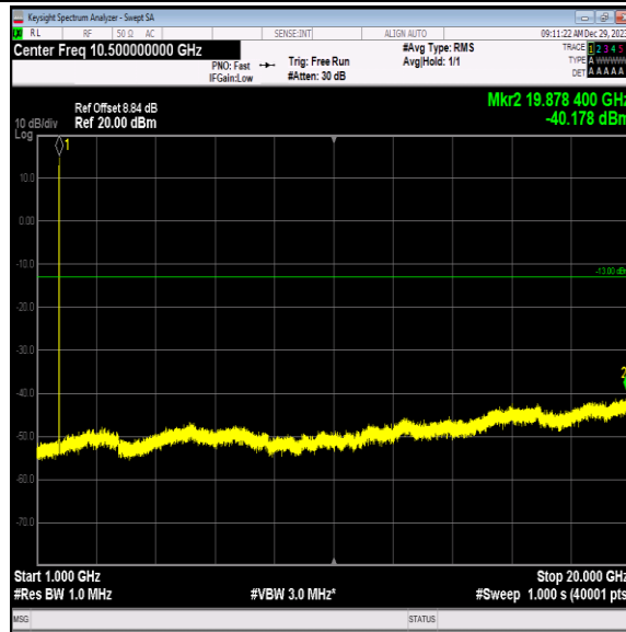
Band4-1312-1-1000~20000MHz-PASS
