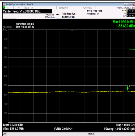
Band4-1312-2-30~1000MHz-PASS
