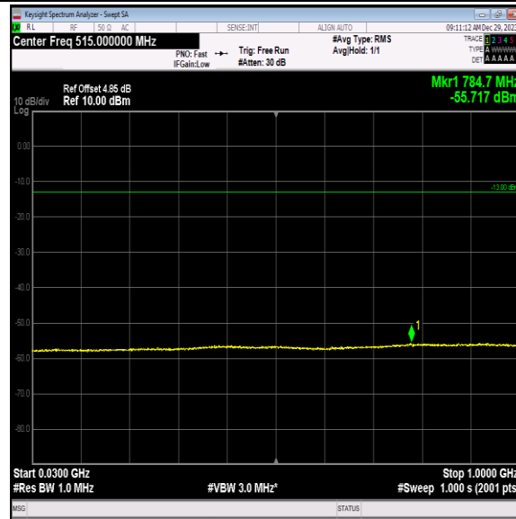
Band4-1312-1-30~1000MHz-PASS
