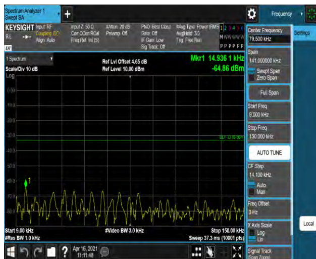
EGPRS850-190-8-0.009~0.15MHz
