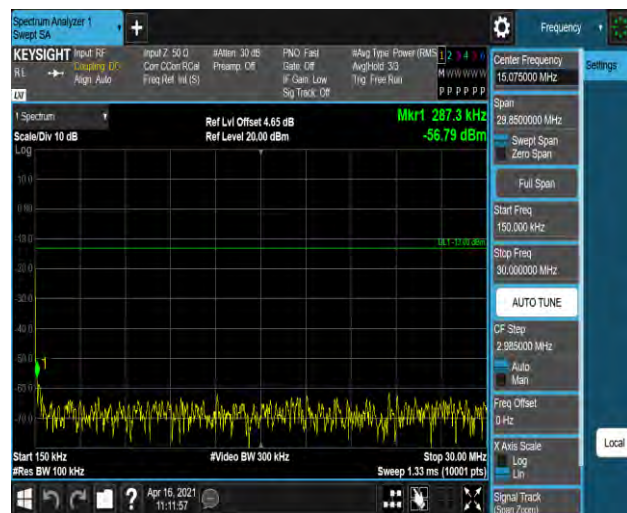
EGPRS850-190-8-0.15~30MHz
