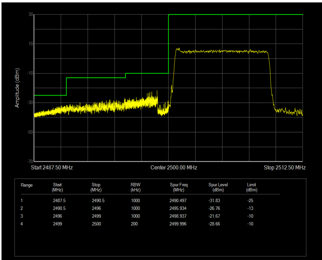
n7 SCS=30kHz CP_QPSK BW=15MHz Channel=501500 RB=1 @37
