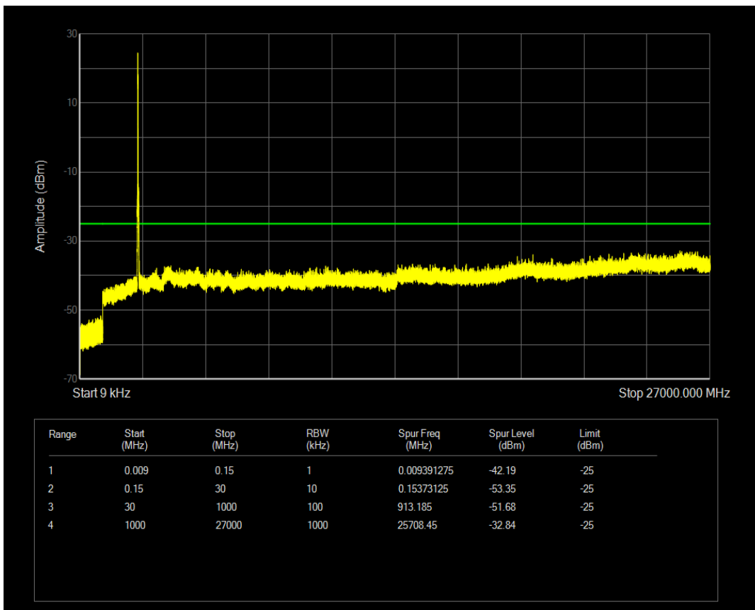
n7 SCS=30kHz CP_QPSK BW=20MHz Channel=512000 RB=1@0
