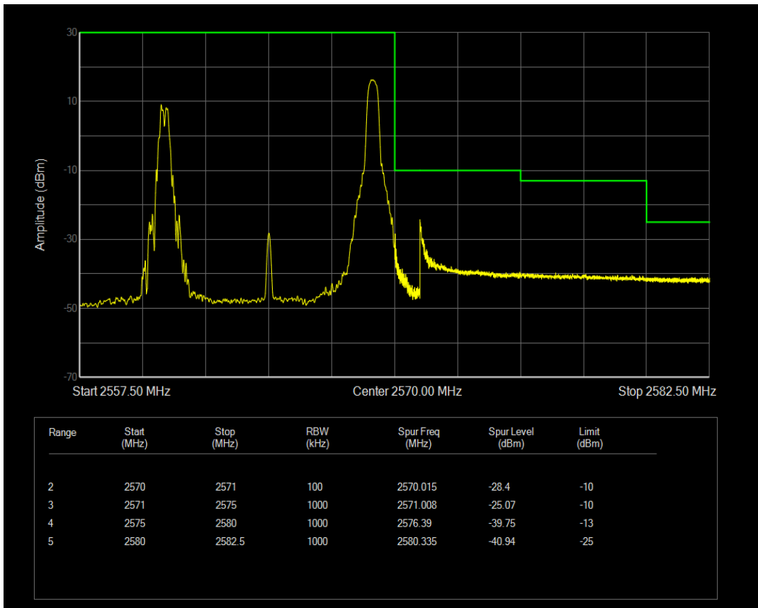
n7 SCS=30kHz CP_QPSK BW=10MHz Channel=513000 RB=1@0
