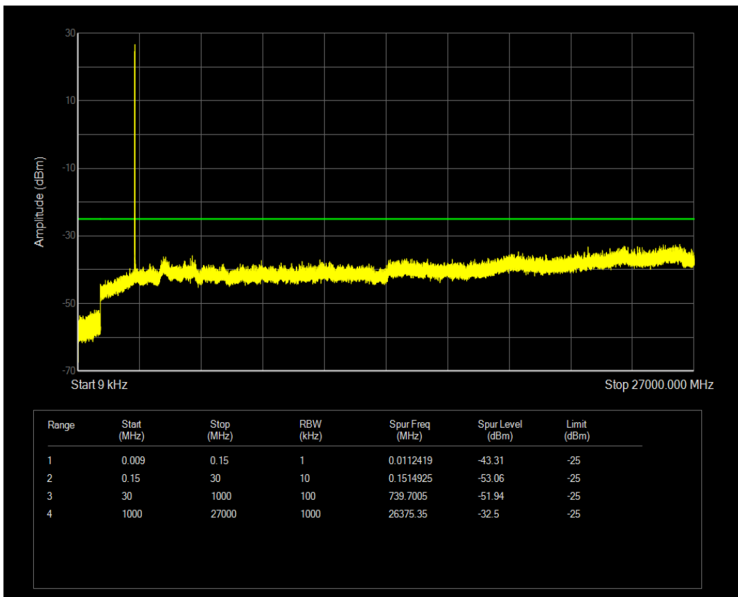
n7 SCS=30kHz CP_QPSK BW=15MHz Channel=501500 RB=38@0
