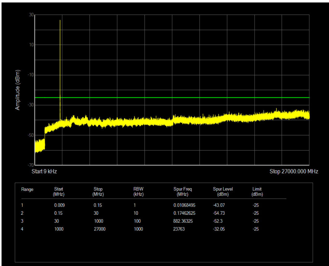
n7 SCS=30kHz CP_QPSK BW=15MHz Channel=501500 RB=1@0
