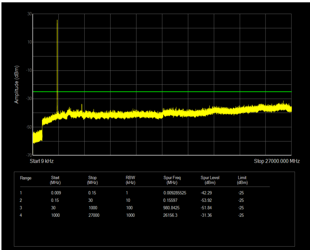
n7 SCS=30kHz CP_QPSK BW=10MHz Channel=513000 RB=24@0
