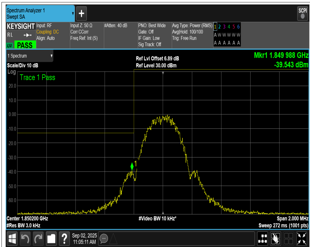
EGPRS1900 Channel=512
