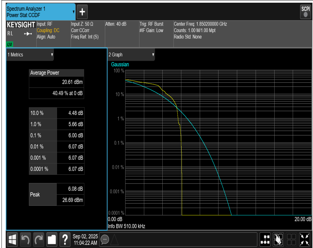
EGPRS1900 Channel=512
