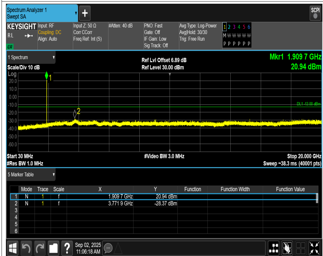
EGPRS1900 Channel=810
