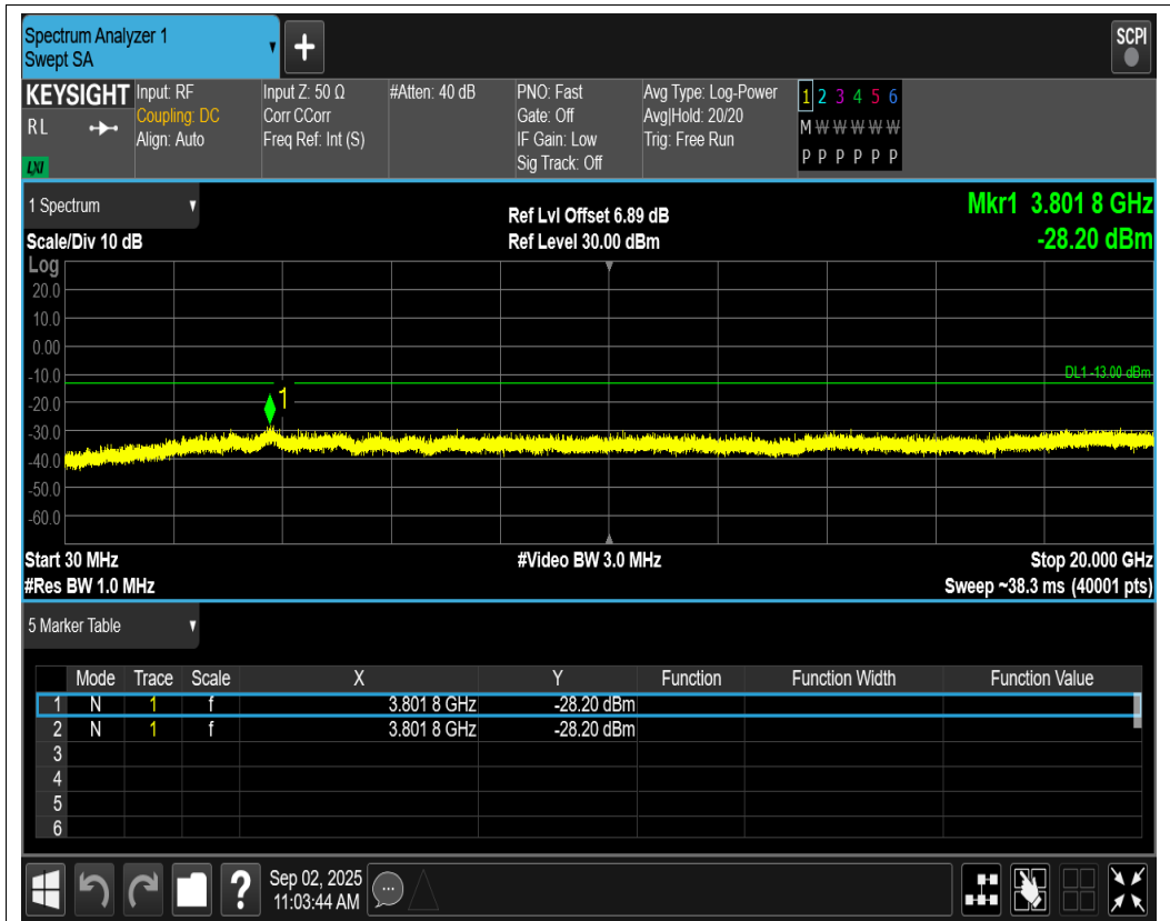
GPRS1900 Channel=810
