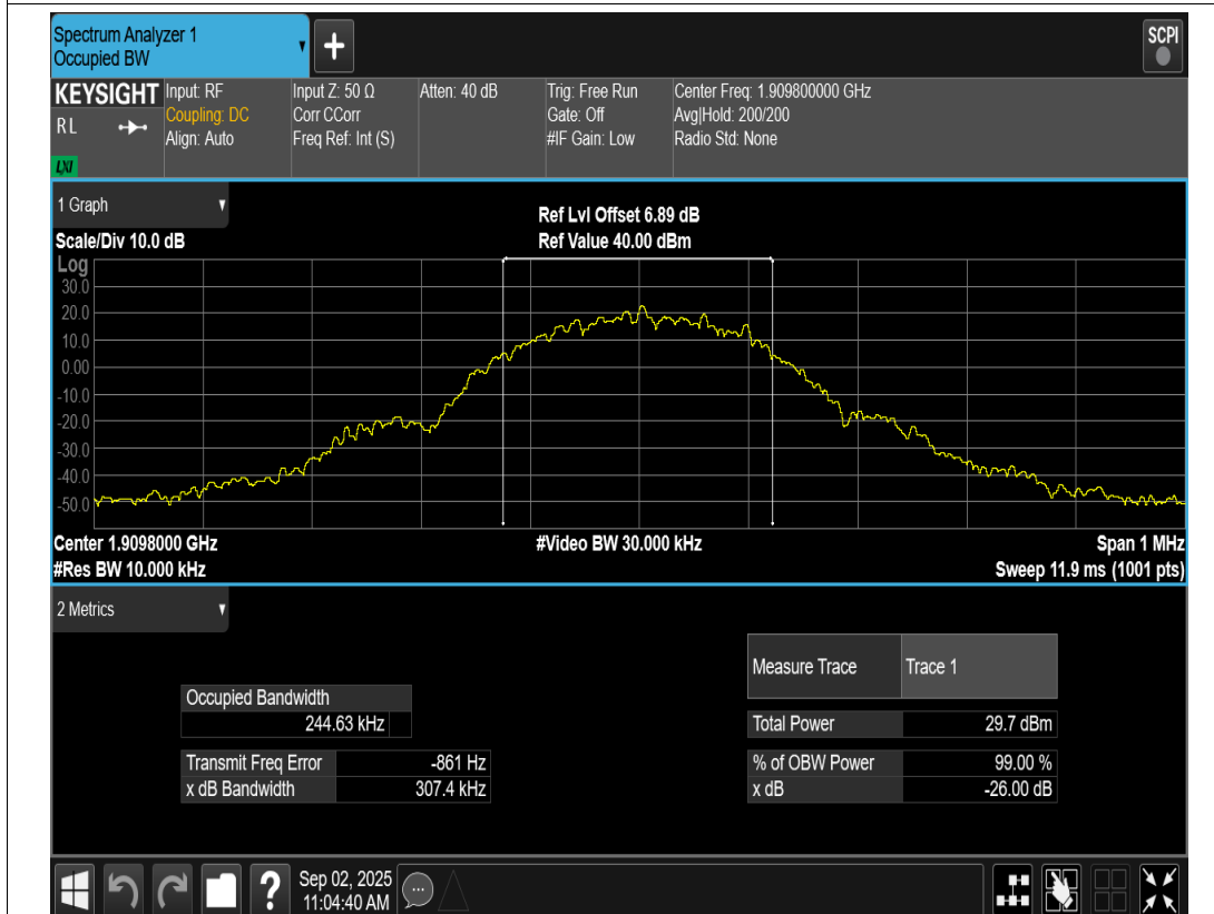
EGPRS1900 Channel=810
