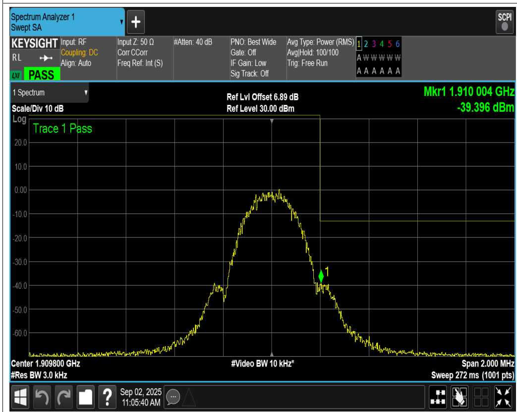
EGPRS1900 Channel=810
