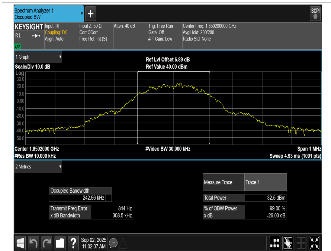
GPRS1900 Channel=512
