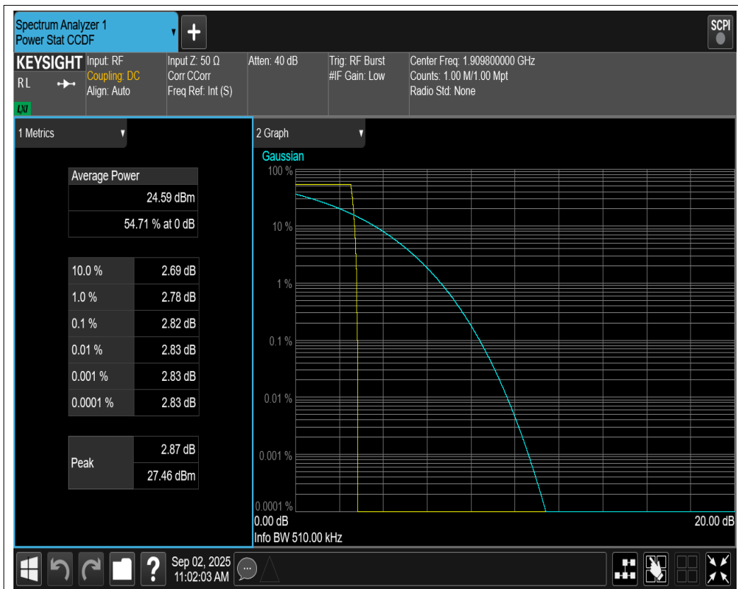
GPRS1900 Channel=810
