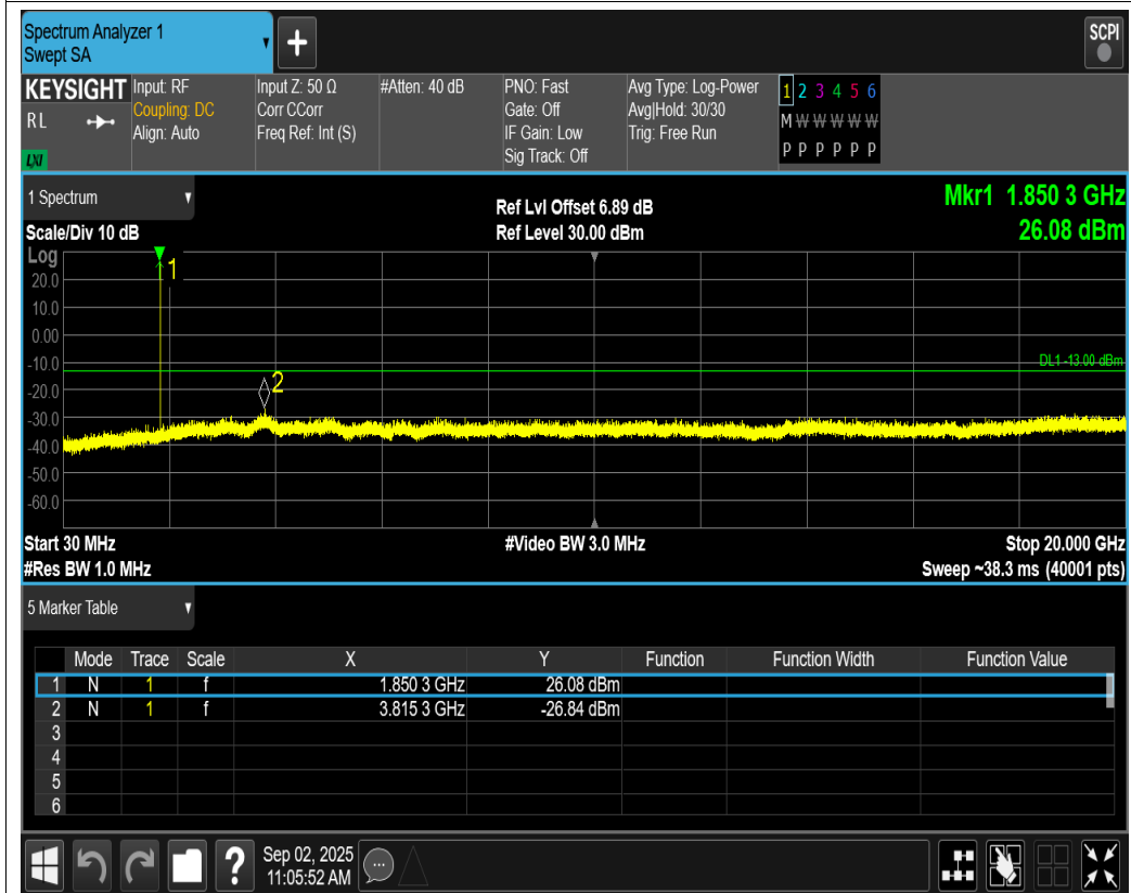
EGPRS1900 Channel=512
