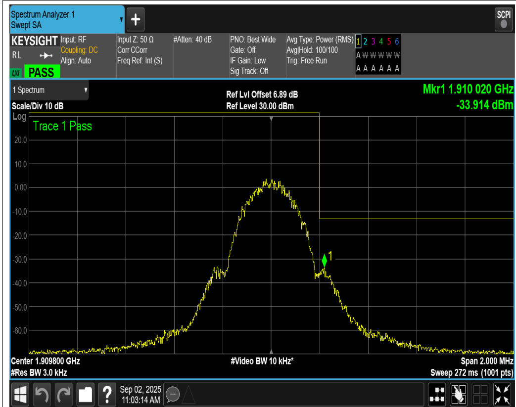
GPRS1900 Channel=810
