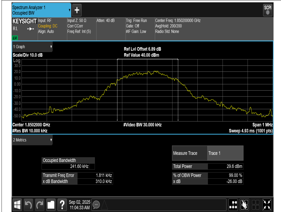
EGPRS1900 Channel=512
