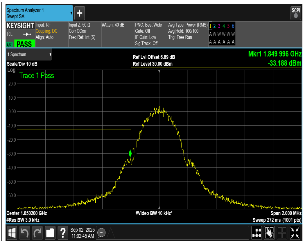
GPRS1900 Channel=512
