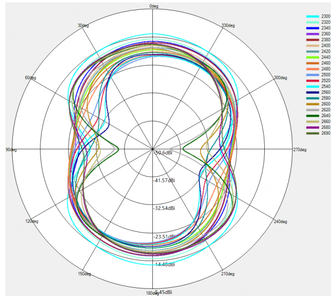
LTE B7/B40/B41 NR n7/n40/n41 \Phi=0^\circ
