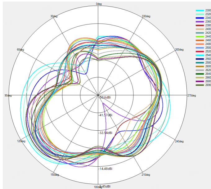
LTE B7/B40/B41 NR n7/n40/n41 \Phi=90^\circ
