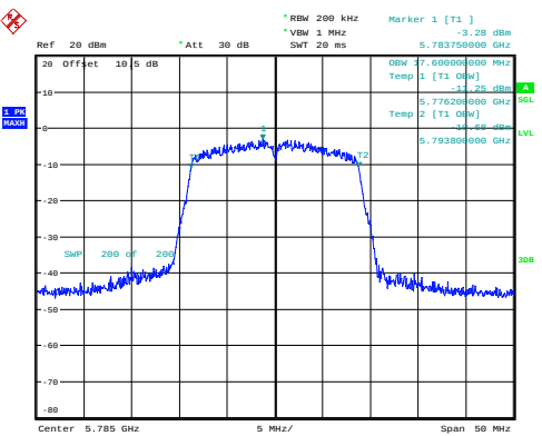
n20_5785MHz_Chain 0 17.600MHz
