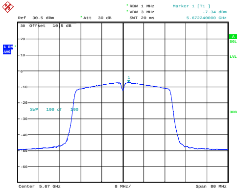
n40_5670MHz_Chain 0 -7.34dBm/MHz
