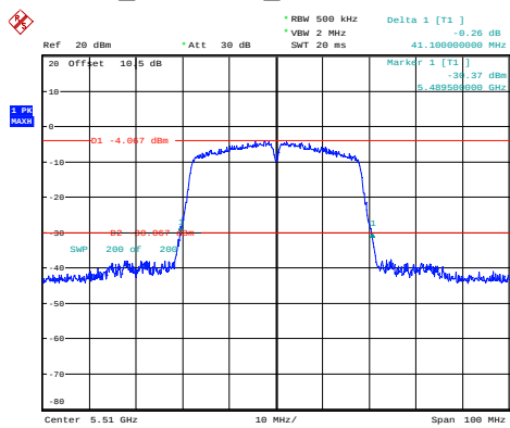
n40_5510MHz_Chain 0 41.100MHz
