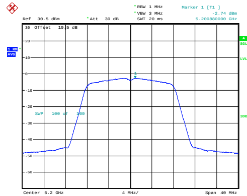
a_5200MHz_Chain 0 -2.74dBm/MHz
