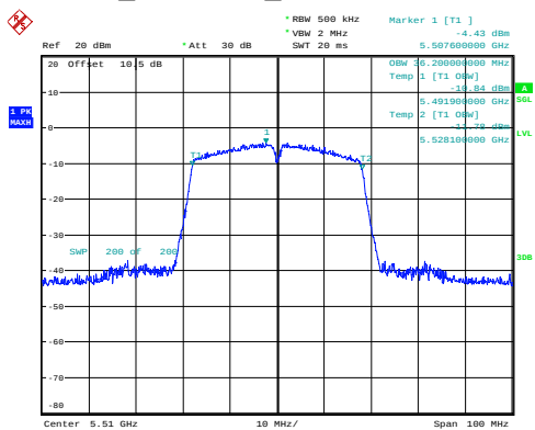
n40_5510MHz_Chain 0 36.200MHz
