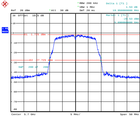
a_5700MHz_Chain 0 19.950MHz
