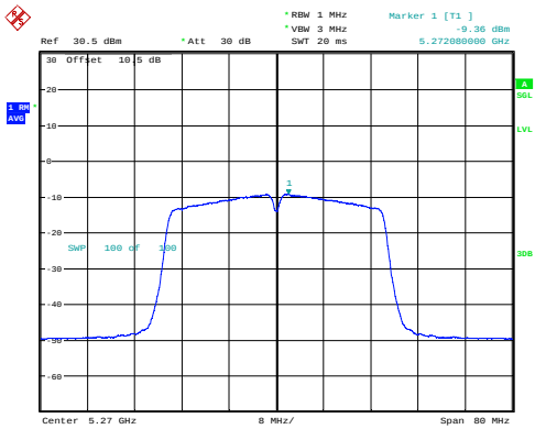
n40_5270MHz_Chain 0 -9.36dBm/MHz
