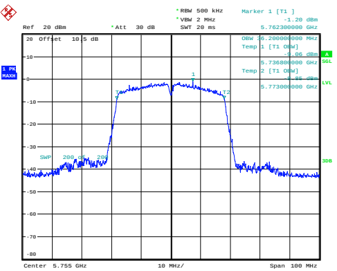
n40_5755MHz_Chain 0 36.200MHz
