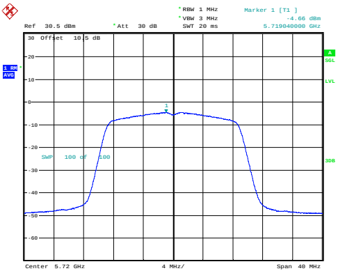
n20_5720MHz_Chain 0 -4.66dBm/MHz
