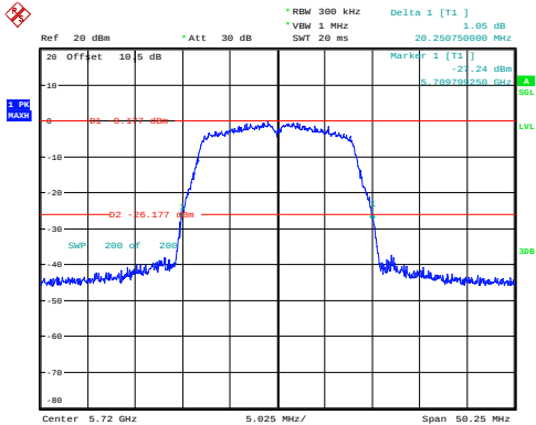
a_5720MHz_Chain 0 20.251MHz
