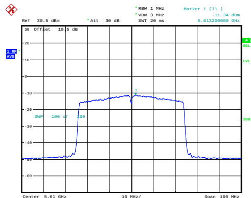
ac80_5610MHz_Chain 0 -11.34dBm/MHz
