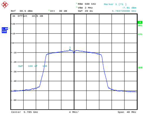
n20_5785MHz_Chain 0 -7.91dBm/MHz
