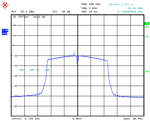
n40_5755MHz_Chain 0 -10.01dBm/MHz
