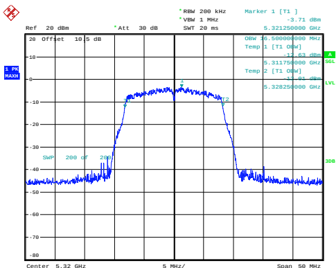
a_5320MHz_Chain 0 16.500MHz
