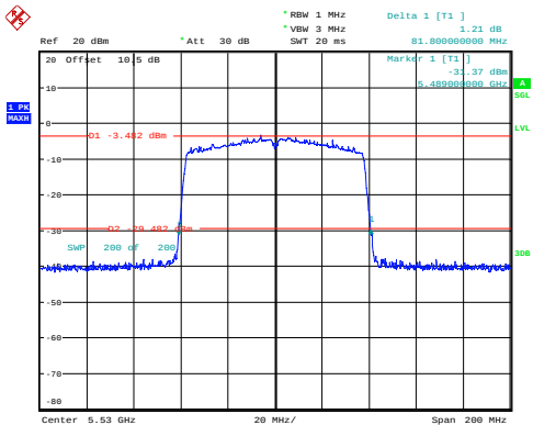
ac80_5530MHz_Chain 0 81.800MHz
