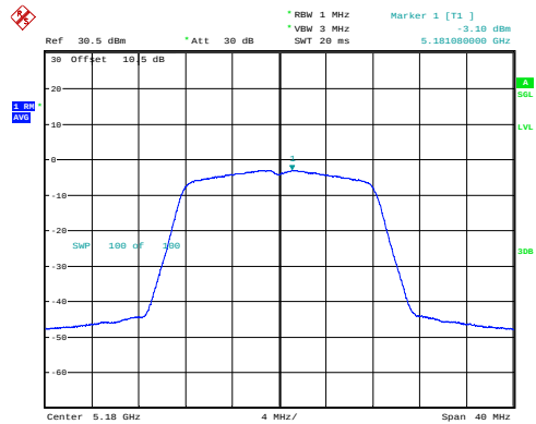
a_5180MHz_Chain 0 -3.08dBm/MHz
