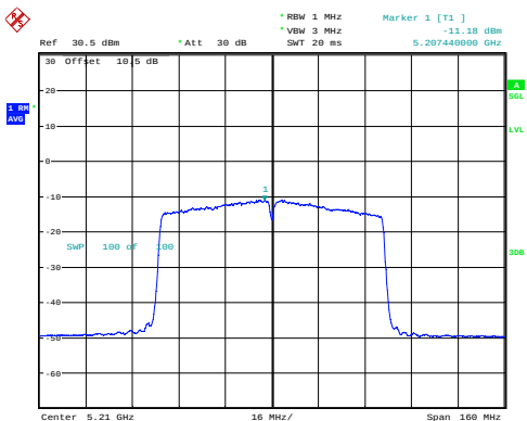
ac80_5210MHz_Chain 0 -11.18dBm/MHz
