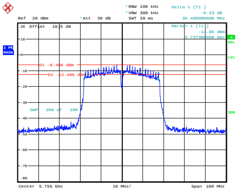
n40_5755MHz_Chain 0 35.400MHz
