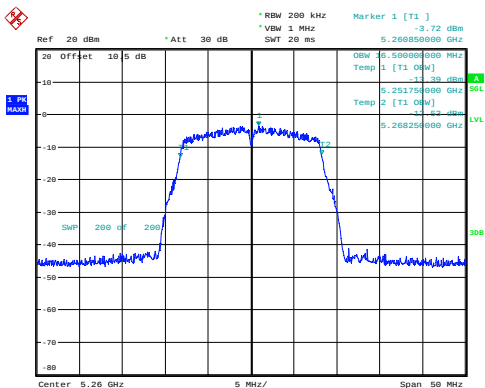
a_5260MHz_Chain 0 16.500MHz
