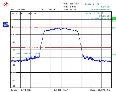
n20_5720MHz_Chain 0 20.655MHz
