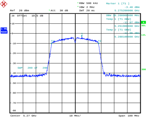
n40_5270MHz_Chain 0 36.200MHz
