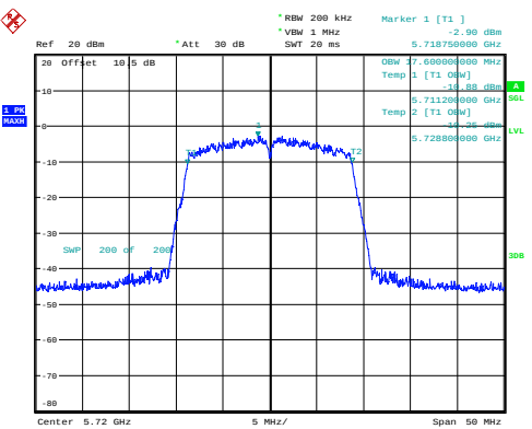
n20_5720MHz_Chain 0 17.600MHz
