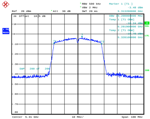
n40_5310MHz_Chain 0 36.200MHz
