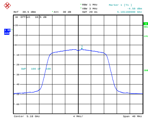
n20_5180MHz_Chain 0 -4.58dBm/MHz
