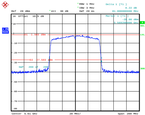
ac80_5610MHz_Chain 0 81.800MHz
