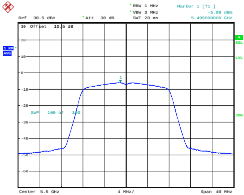
a_5500MHz_Chain 0 -5.98dBm/MHz
