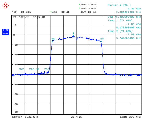
ac80_5210MHz_Chain 0 75.400MHz
