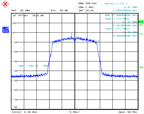
n20_5260MHz_Chain 0 17.600MHz
