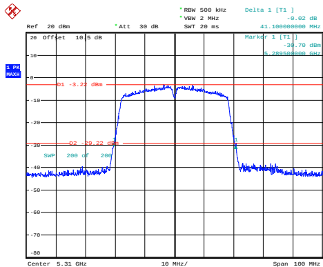
n40_5310MHz_Chain 0 41.100MHz
