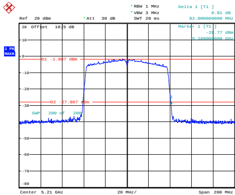
ac80_5210MHz_Chain 0 82MHz
