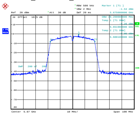
n40_5670MHz_Chain 0 36.200MHz
