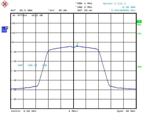
a_5580MHz_Chain 0 -4.38dBm/MHz
