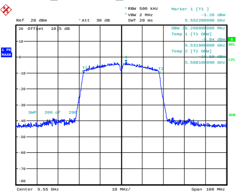
n40_5550MHz_Chain 0 36.200MHz
