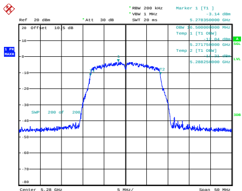
a_5280MHz_Chain 0 16.500MHz
