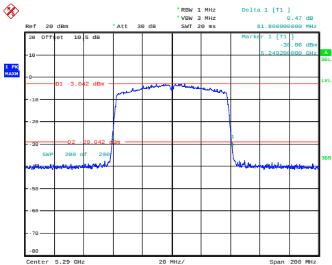
ac80_5290MHz_Chain 0 81.800MHz
