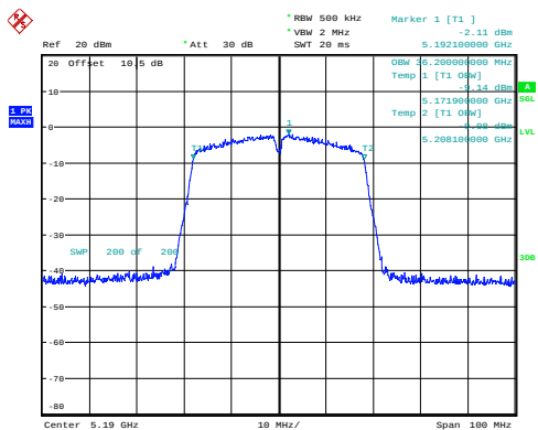
n40_5190MHz_Chain 0 36.200MHz
