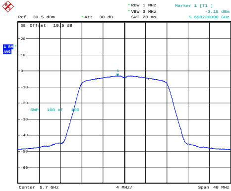
a_5700MHz_Chain 0 -3.15dBm/MHz
