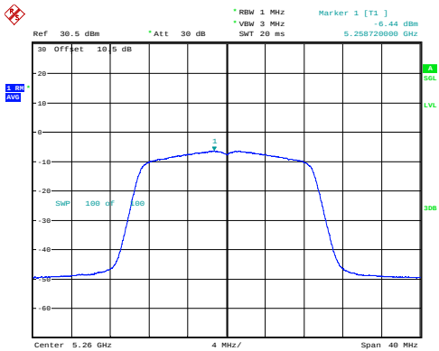
n20_5260MHz_Chain 0 -6.44dBm/MHz
