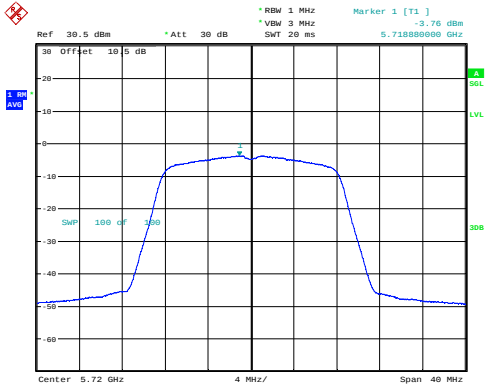
a_5720MHz_Chain 0 -3.76dBm/MHz
