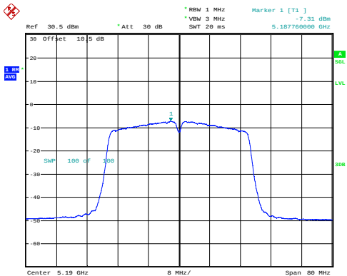
n40_5190MHz_Chain 0 -7.31dBm/MHz
