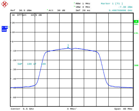
n20_5500MHz_Chain 0 -7.30dBm/MHz
