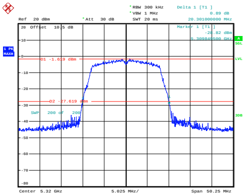
a_5320MHz_Chain 0 20.301MHz
