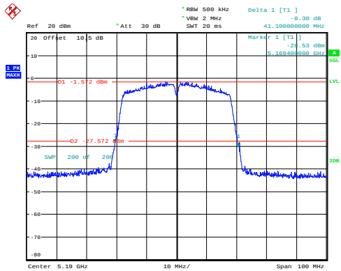
n40_5190MHz_Chain 0 41.100MHz
