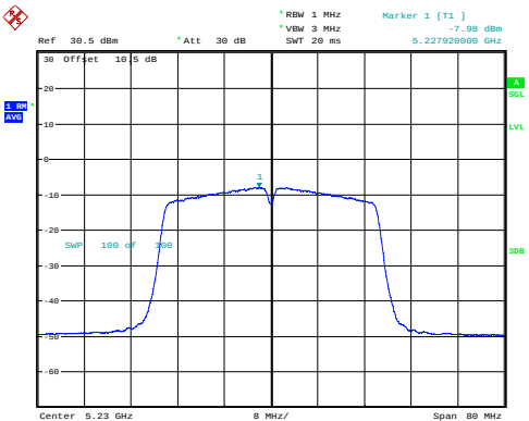
n40_5230MHz_Chain 0 -7.98dBm/MHz
