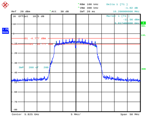
a_5825MHz_Chain 0 15.200MHz
