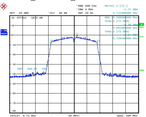
n40_5710MHz_Chain 0 36.200MHz
