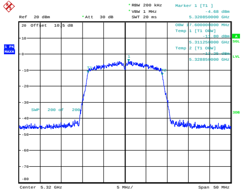
n20_5320MHz_Chain 0 17.600MHz
