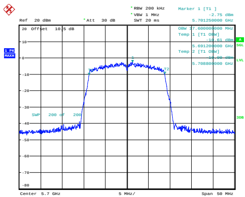
n20_5700MHz_Chain 0 17.600MHz
