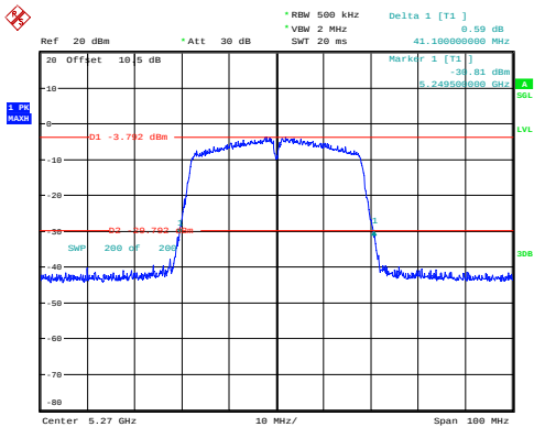
n40_5270MHz_Chain 0 41.100MHz
