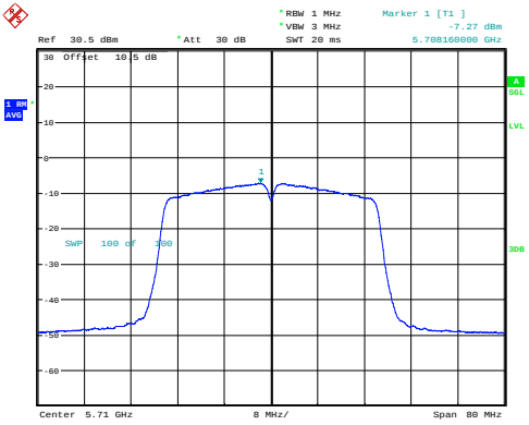
n40_5710MHz_Chain 0 -7.27dBm/MHz
