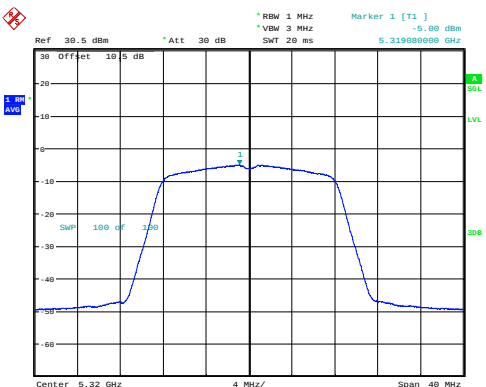
a_5320MHz_Chain 0 -5.00dBm/MHz
