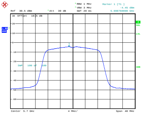
n20_5700MHz_Chain 0 -4.45dBm/MHz
