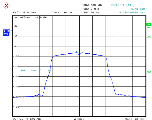
a_5785MHz_Chain 0 -6.48dBm/MHz
