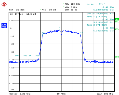
n40_5230MHz_Chain 0 36.200MHz
