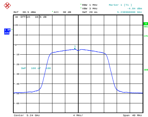
n20_5240MHz_Chain 0 -4.84dBm/MHz
