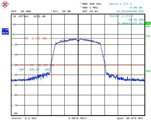
n20_5500MHz_Chain 0 20.655MHz
