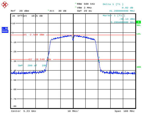
n40_5230MHz_Chain 0 41.200MHz
