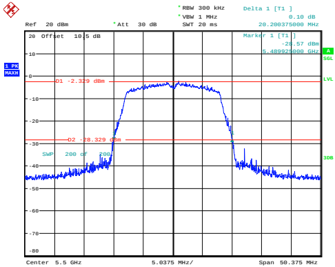
a_5500MHz_Chain 0 20.200MHz
