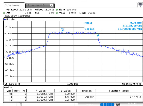
n20_5320MHz_Chain 0
