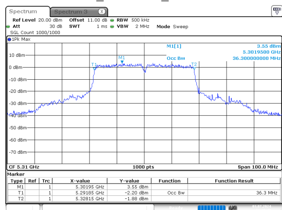
n40_5310MHz_Chain 0
