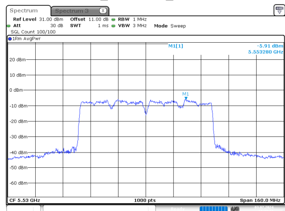
ac80_5530MHz_Chain 0
