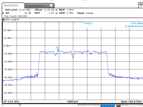
ac80_5610MHz_Chain 0
