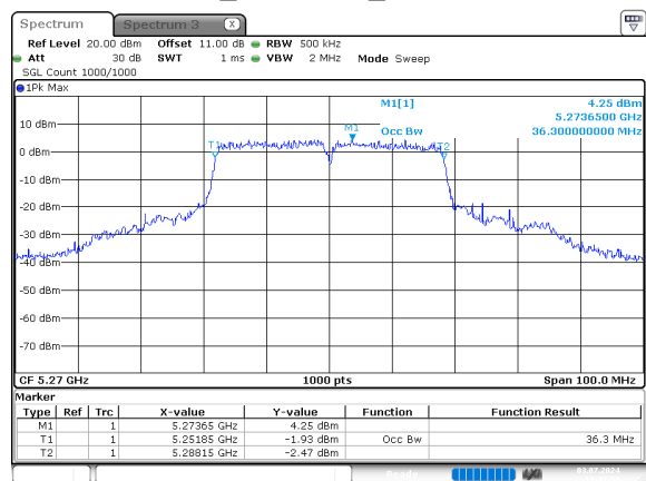
n40_5270MHz_Chain 0
