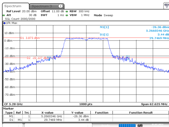
a_5280MHz_Chain 0
