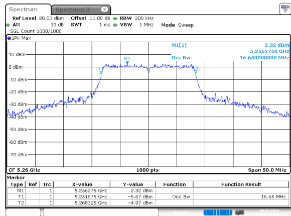
a_5260MHz_Chain 0
