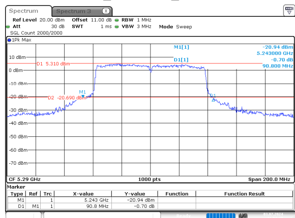
ac80_5290MHz_Chain 0
