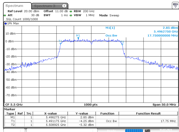
n20_5500MHz_Chain 0
