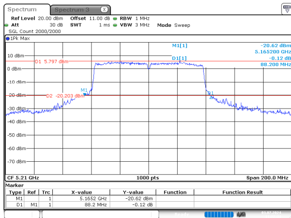
ac80_5210MHz_Chain 0
