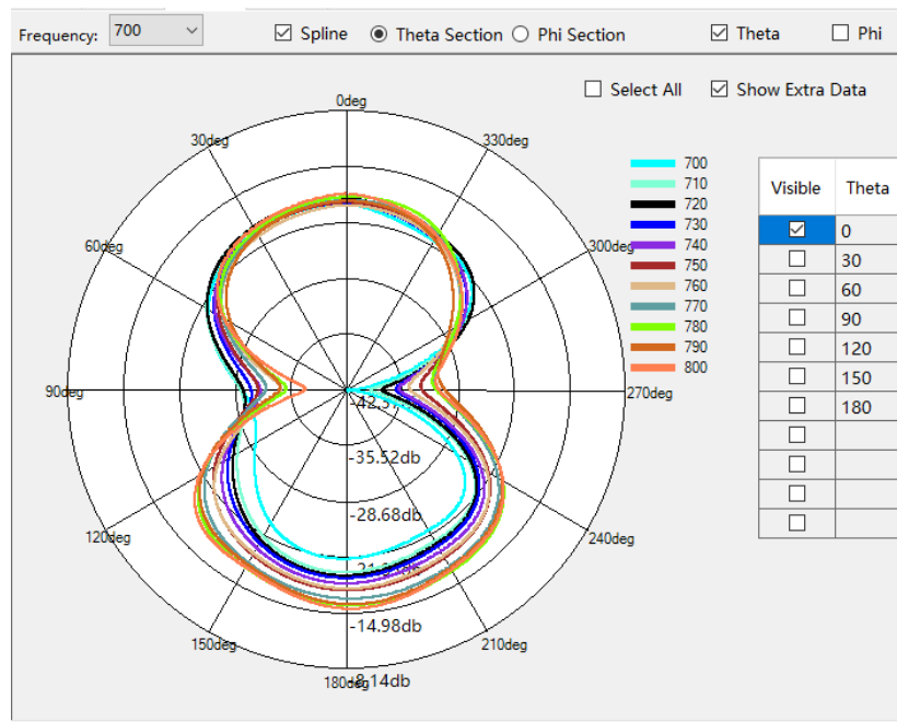
LTE B12/17/28 NR n12/n17/n28 Phi=0deg
