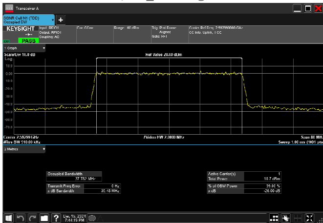
n41_50MHz_30kHz_2592.99MHz_DFT-s-OFDM QPSK_RB128@0
