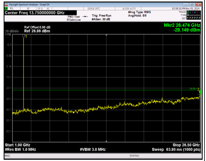
Band7-5MHz-16QAM-21425-1RB#0-Range2:1000~26 500MHz
