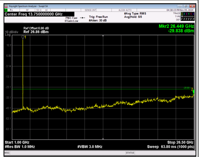
Band7-20MHz-QPSK-21100-1RB#0-Range2:1000~26 500MHz
