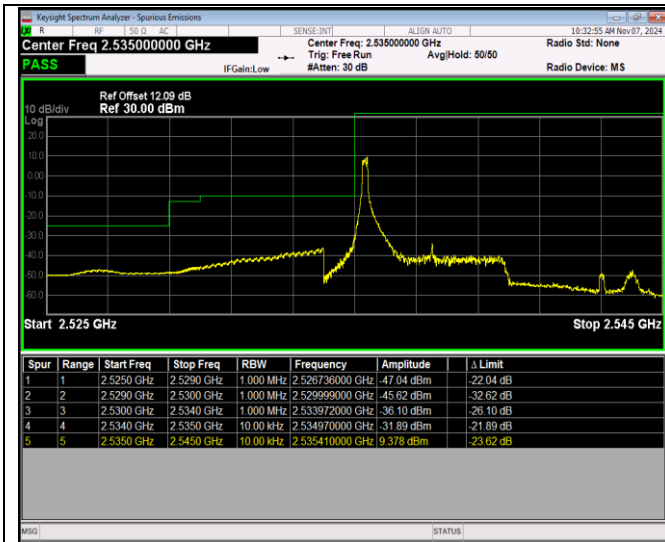
Band41-5MHz-QPSK-40065-25RB#0
