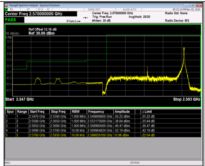
Band38-20MHz-QPSK-38150-1RB#0
