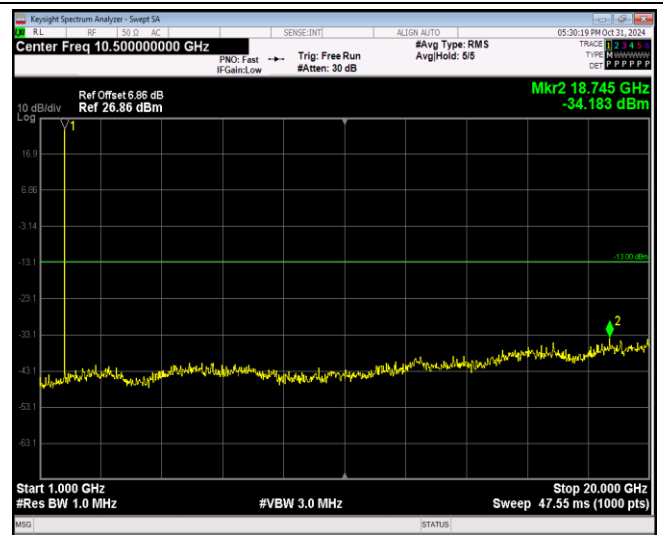
Band66-20MHz-QPSK-132072-1RB#0-Range2:1000~20000MHz
