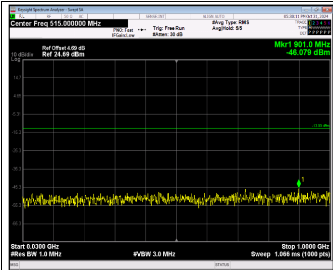
Band66-20MHz-QPSK-132072-1RB#0-Range1:30~1000MHz
