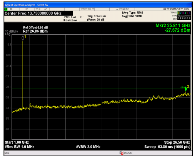
Band38-5MHz-QPSK-38000-1RB#0-Range2:1000~2 6500MHz
