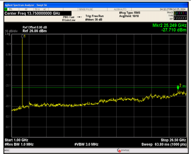
Band38-5MHz-QPSK-38000-1RB#0-Range2:1000~2 6500MHz
