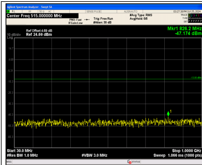
Band4-20MHz-QPSK-20175-1RB#0-Range1:30~100 0MHz
