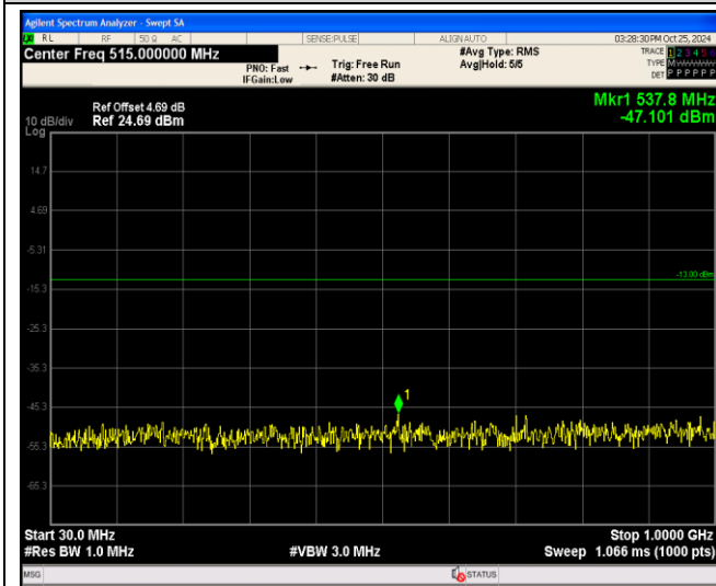
Band4-20MHz-QPSK-20300-1RB#0-Range1:30~100 0MHz
