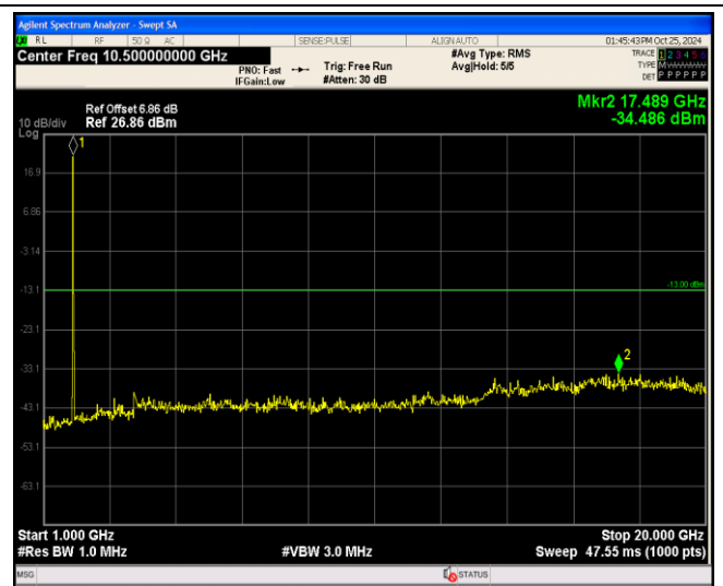
Band2-20MHz-16QAM-18900-1RB#0-Range2:1000~20000MHz
