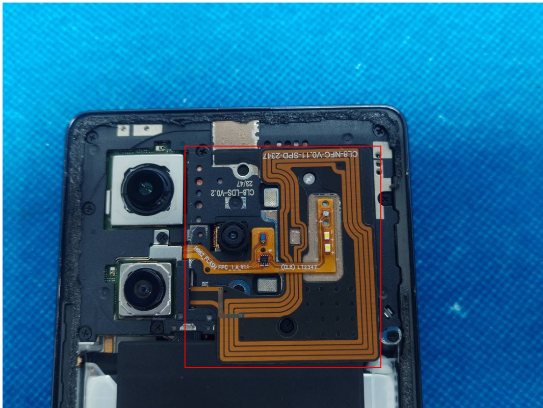
NFC ANT
