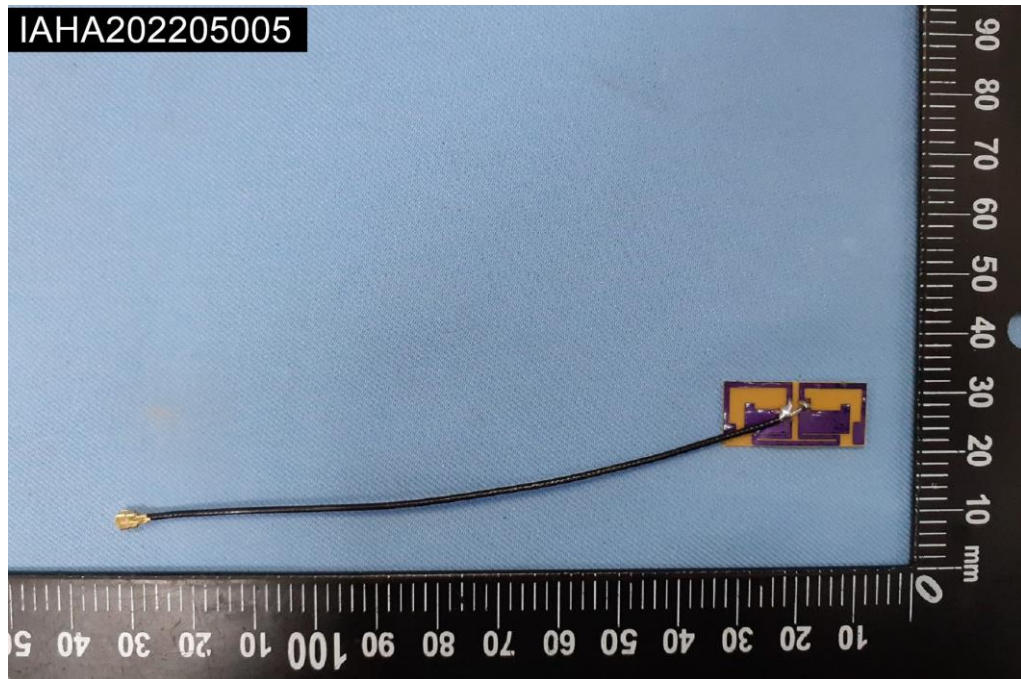
EUT Photo (12)
