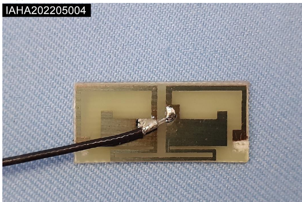
EUT Photo (8)
