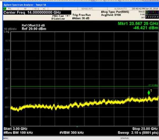
3GHz-25GHz
