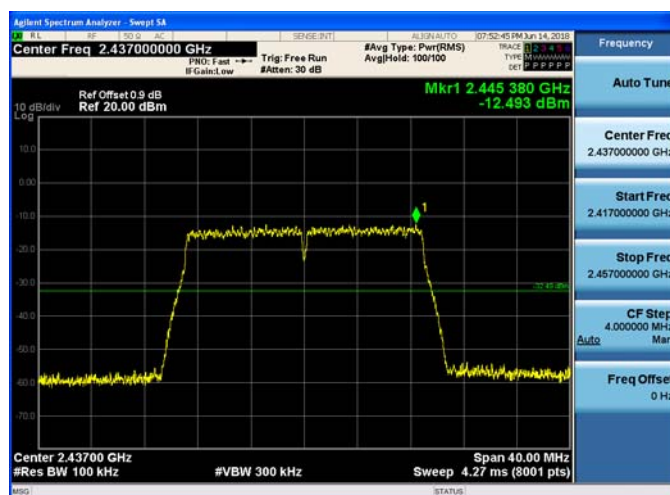
802.11n(HT20) CH06
