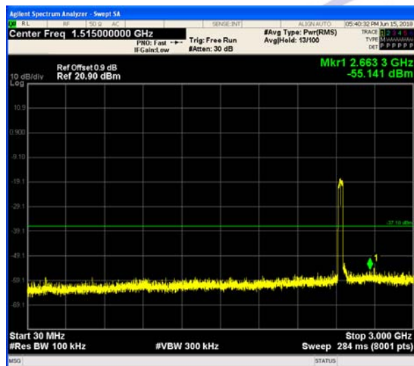
30MHz-3GHz
