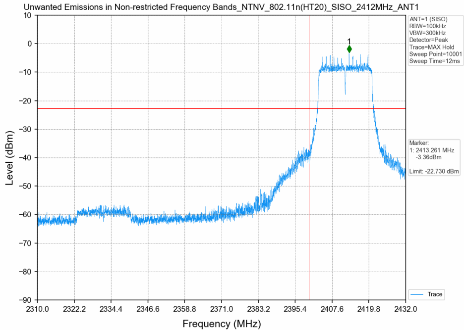
802.11n(HT20)_2412MHz_SISO_ANT1
