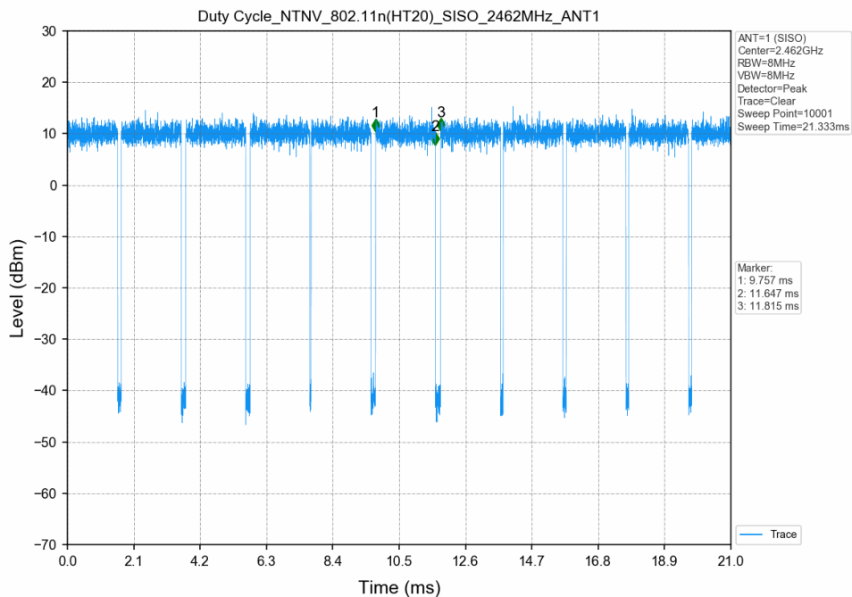
802.11n(HT20)_2462MHz_SISO_ANT1
