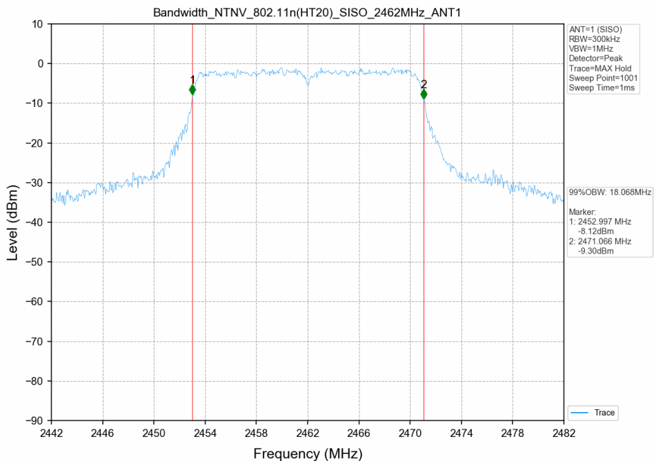
802.11n(HT20)_2462MHz_SISO_ANT1
