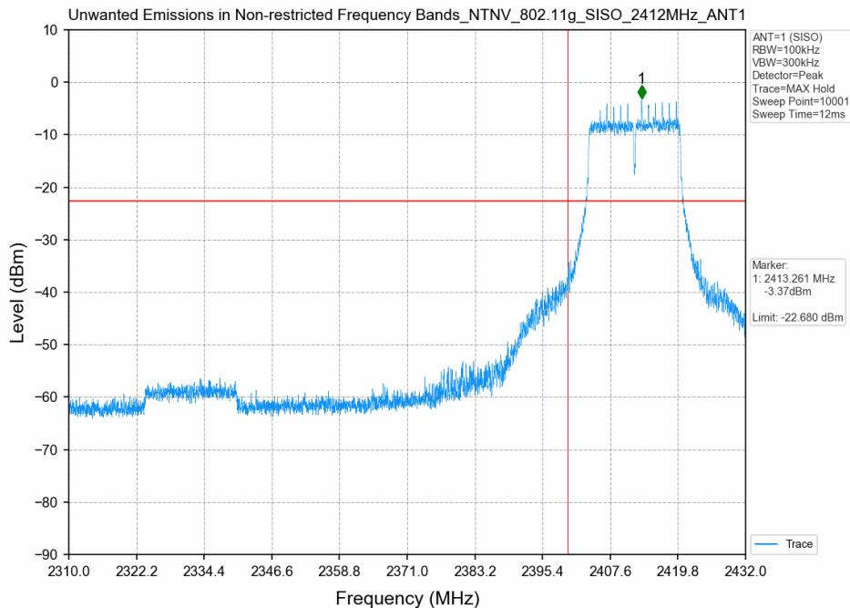
802.11g_2412MHz_SISO_ANT1
