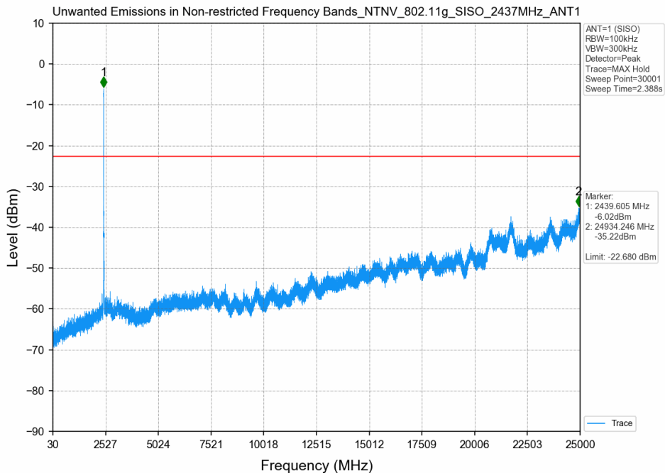
802.11g_2437MHz_SISO_ANT1
