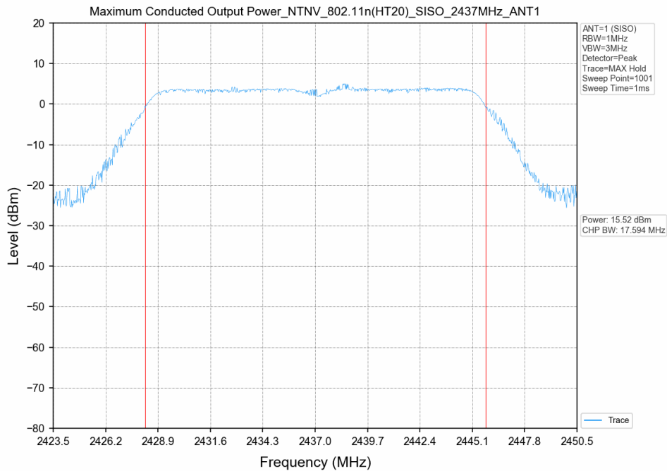
802.11n(HT20)_2437MHz_SISO_ANT1
