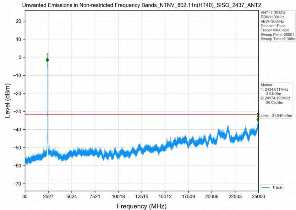
802.11n(HT40)_2437MHz_SISO_ANT2
