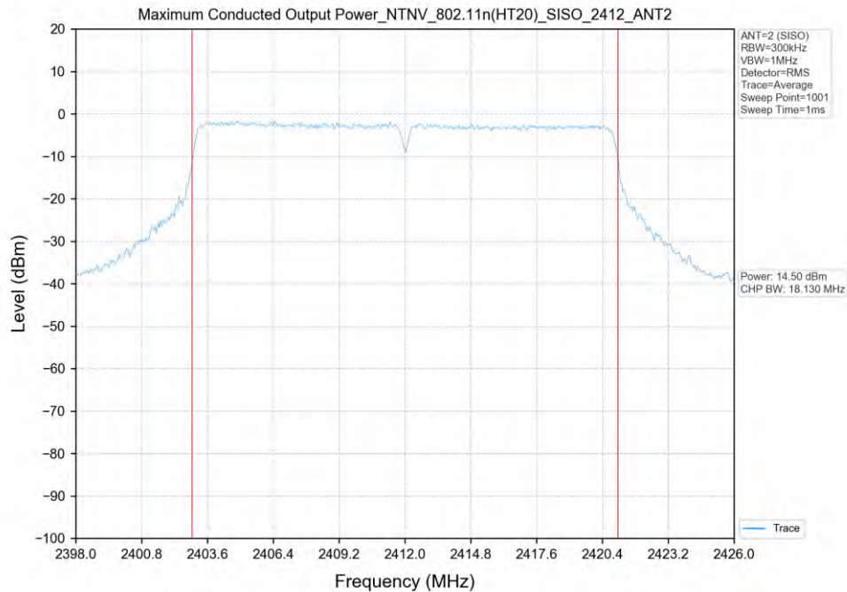
802.11n(HT20)_2412MHz_SISO_ANT2
