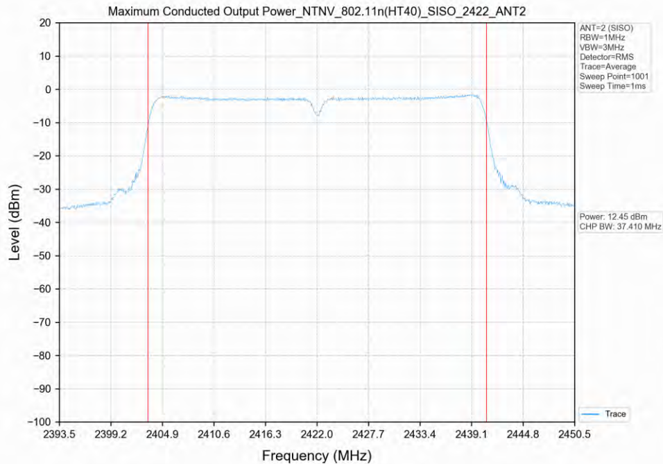
802.11n(HT40)_2422MHz_SISO_ANT2
