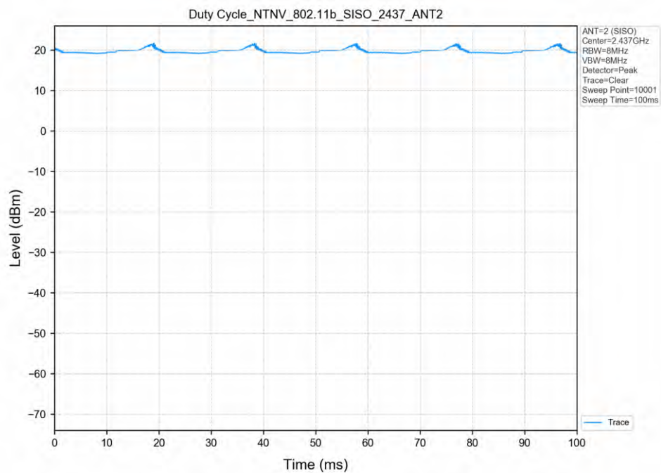
802.11b_2437MHz_SISO_ANT2
