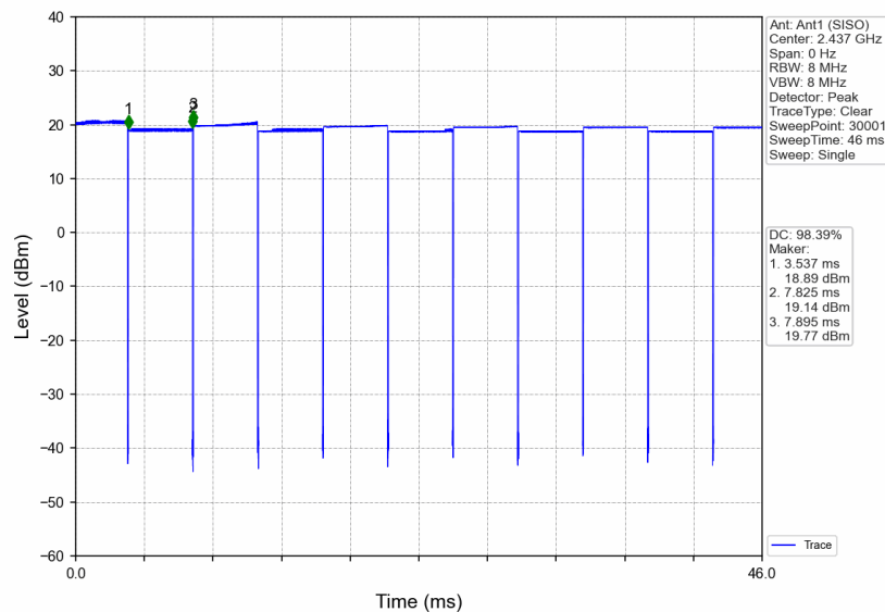
802.11b_MCH_2437MHz_Ant1 (SISO)_NTNV
