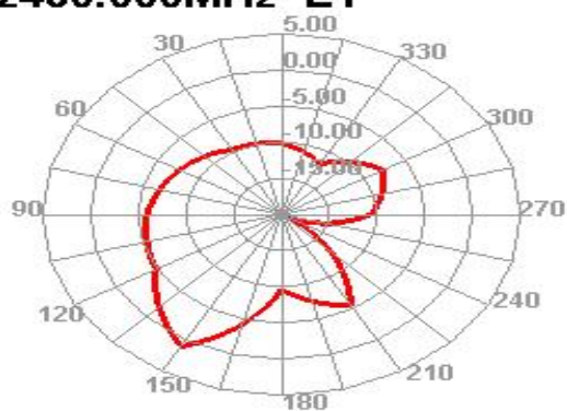
2480.000MHz E1
