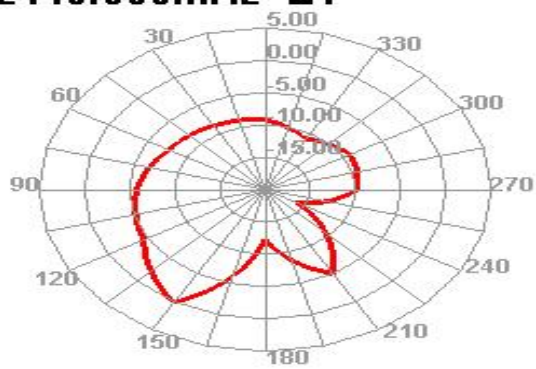
2440.000MHz E1
