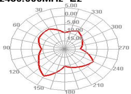
2480.000MHz E2
