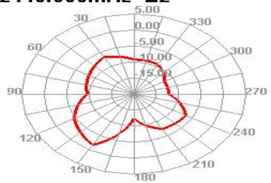
2440.000MHz E2
