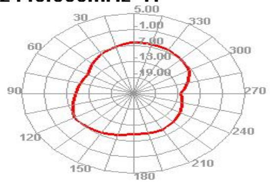
2440.000MHz E2
