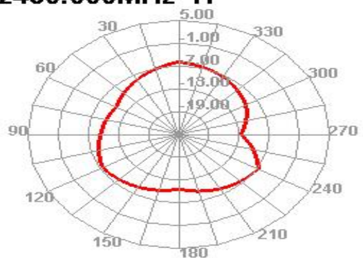
2480.000MHz H
