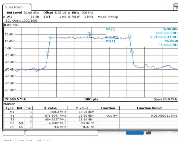
n71 SCS=15kHz DFT_BPSK BW=10MHz Channel=136100 RB=50@0
