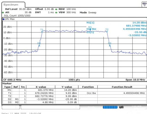
n71 SCS=15kHz CP_16QAM BW=5MHz Channel=136100 RB=25@0
