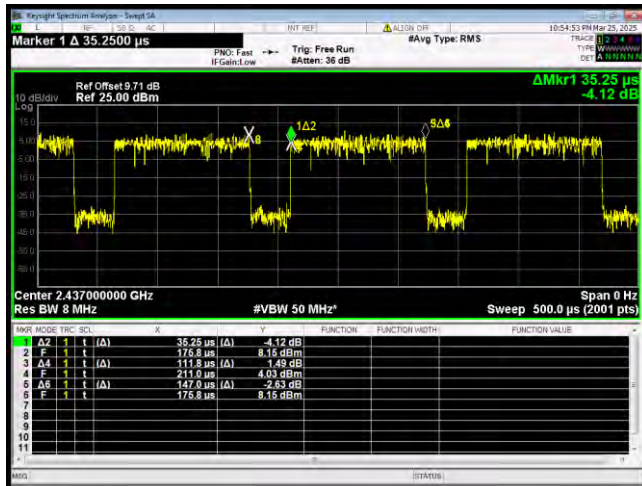
802.11g 2437MHz
