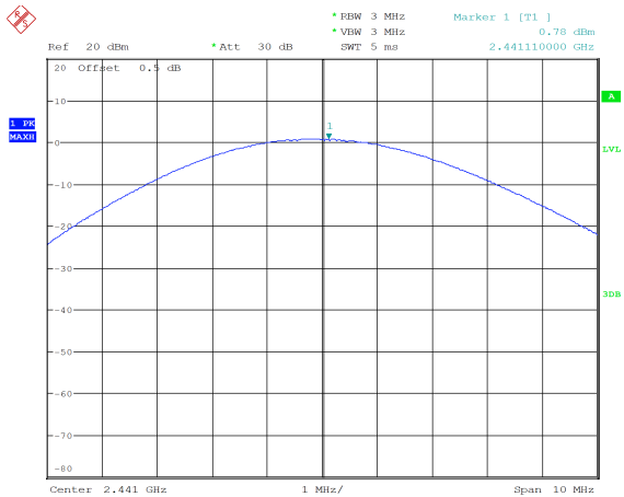
\pi/4 -DQPSK_Middle 0.78 dBm
