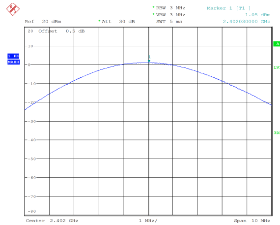
\pi/4 -DQPSK_Low 1.05 dBm
