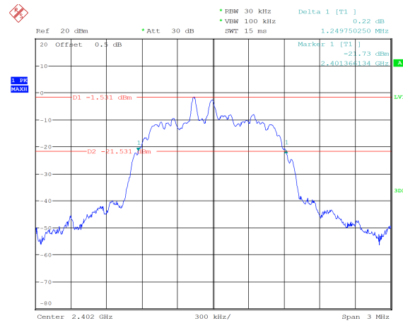
\pi/4 -DQPSK_Low 1.250 MHz
