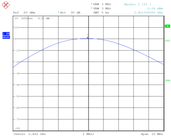
GFSK_Low 0.24 dBm
