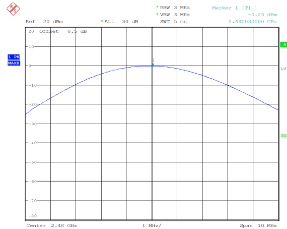
\pi/4 -DQPSK_High -0.23 dBm
