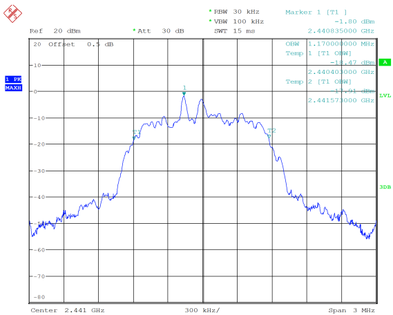
\pi/4 -DQPSK_Middle 1.170 MHz
