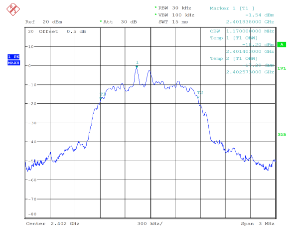
\pi/4 -DQPSK_Low 1.170 MHz
