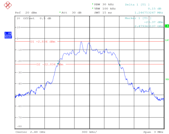
\pi/4 -DQPSK_High 1.247 MHz
