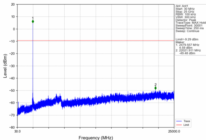
Zigbee_HCH_2480MHz_Ant1_NTNV
