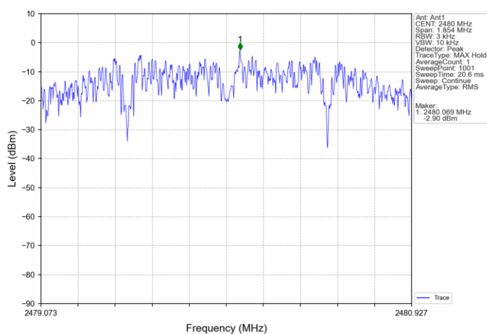
Zigbee_HCH_2480MHz_Ant1_NTNV
