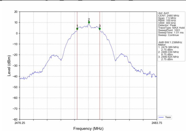
Zigbee_HCH_2480MHz_Ant1_NTNV
