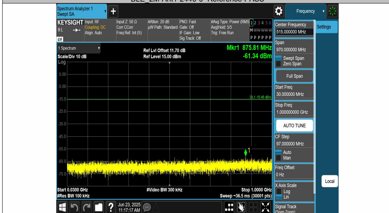
BLE_2M-Ant1-2440-30~1000-PASS
