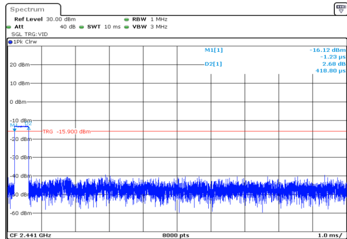
DH1_Ant1_Hop
