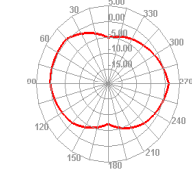
Bluetooth 0 TRP E2
