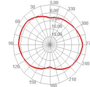
Bluetooth 39 TRP E2
