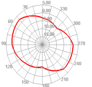
Bluetooth 39 TRP E1
