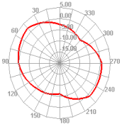
Bluetooth 78 TRP E1
