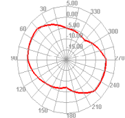
Bluetooth 0 TRP E1
