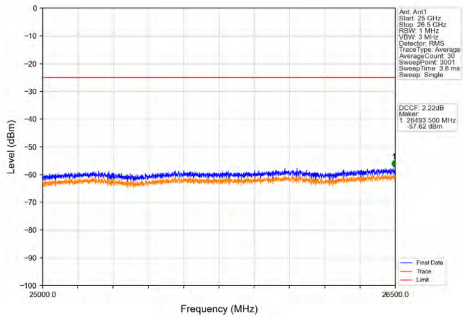
Band41_20MHz_QPSK_HCH_2680MHz_RB_1_99_NTNV
