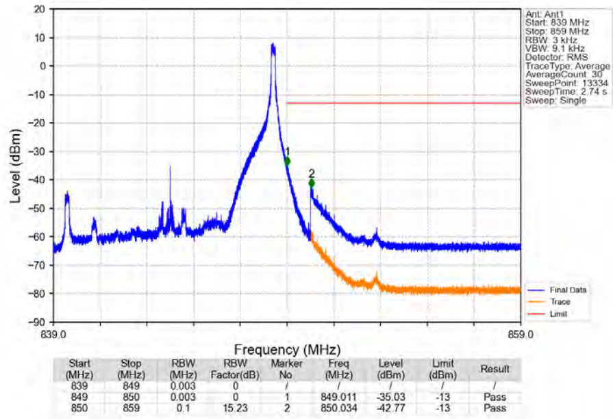
Band26b_10MHz_QPSK_HCH_844MHz_RB_1_49_NTNV
