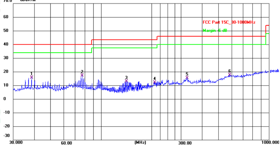
Horizontal 70.0 dBuV/m
