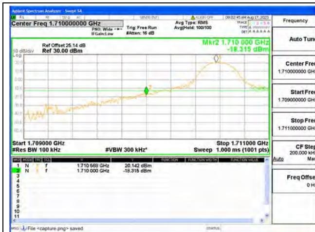
B66 / 10MHz / Low CH / QPSK / 1 RB
