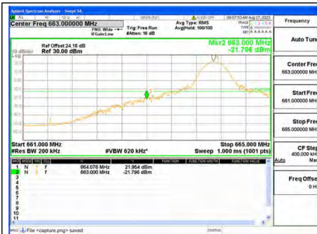
B71 / 20MHz / Low CH / QPSK / 1 RB
