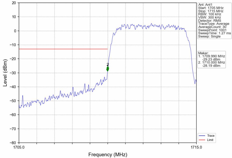
Band4_HSUPA_LCH_1712.4MHz_Subtest 1_NTNV
