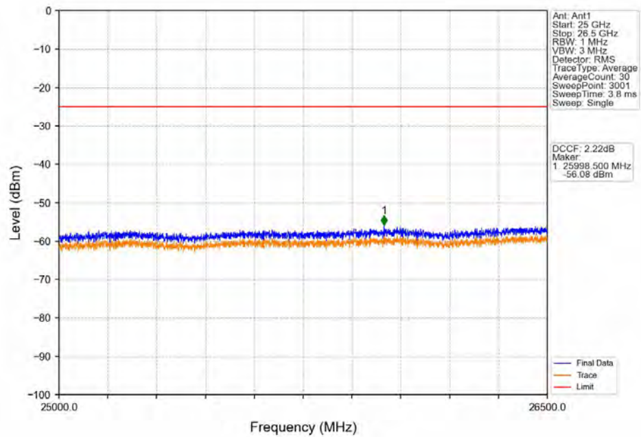
Band41_20MHz_QPSK_MCH_2600MHz_RB_1_0_NTNV
