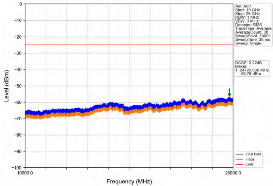
Band41_15MHz_QPSK_LCH_2557.5MHz_RB_1_0_NTNV
