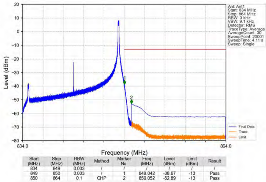
Band26b_15MHz_QPSK_HCH_841.5MHz_RB_1_74_NTNV
