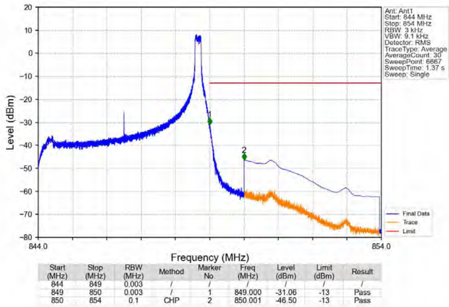
Band5_5MHz_QPSK_HCH_846.5MHz_RB_1_24_NTNV
