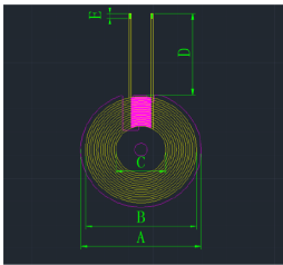
一、尺寸 DIMENSION:(mm)
