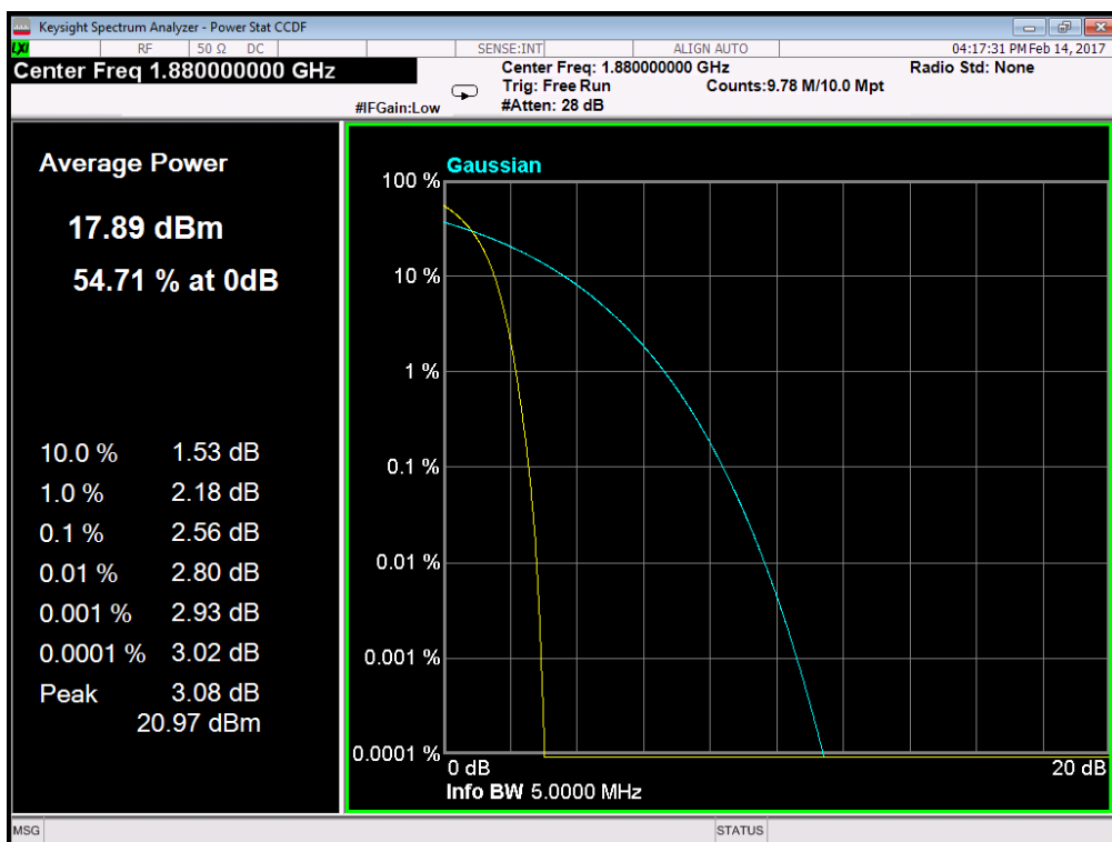
(Plot A2: WCDMA 1900MHz Channel = 9400)
