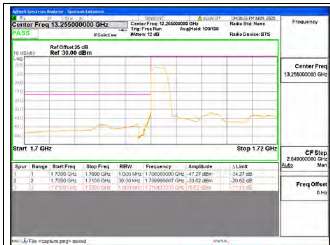
B4 / 10MHz / Low CH / QPSK / 1 RB
