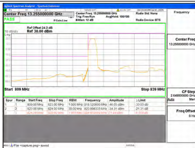
B26 / 15MHz / Low CH / QPSK / 1 RB
