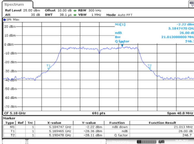
ANT 1(11A)
