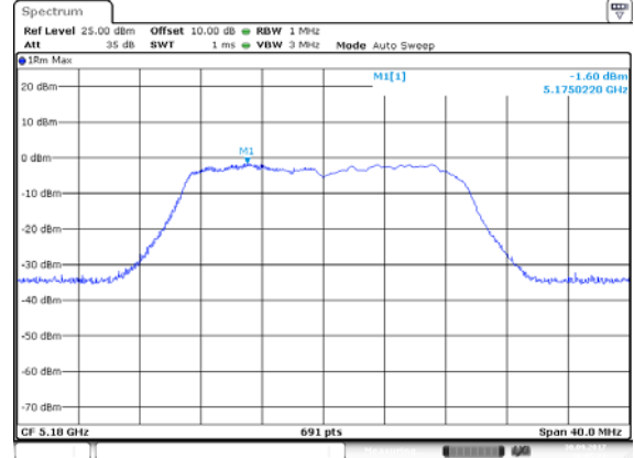
ANT 2(11AC20)
