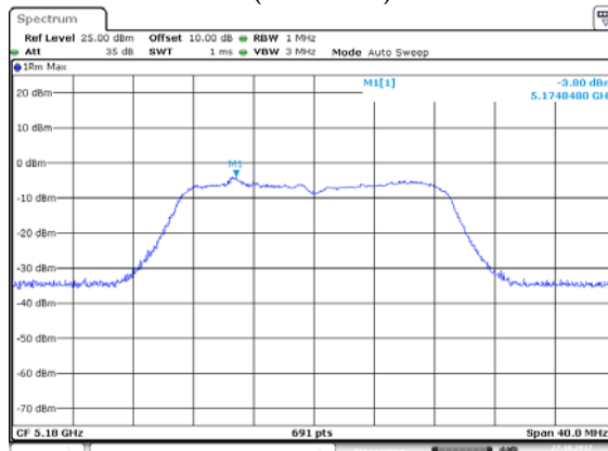
ANT 2(11AC20)
