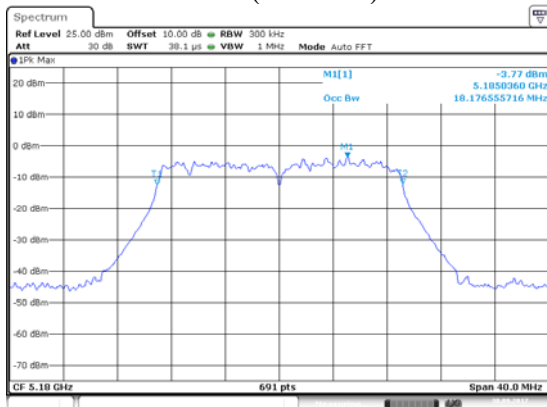
ANT 1(11AC20)
