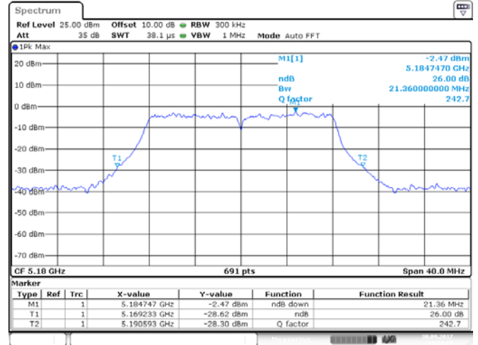
ANT 2(11A)
