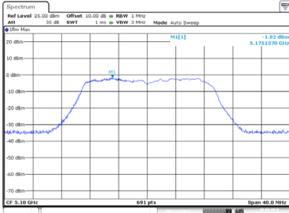
ANT 1(11AC20)
