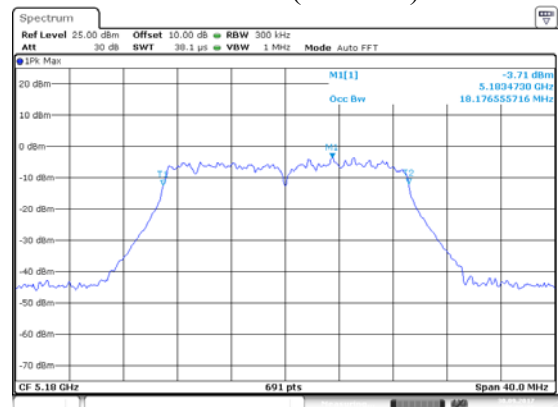
ANT 2(11AC20)
