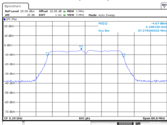
ANT 1(11N40)
