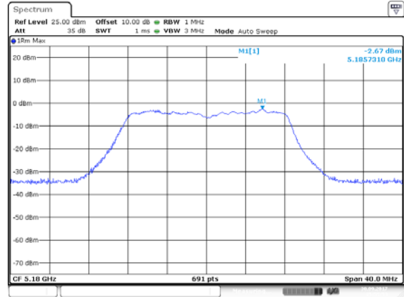
ANT 2(11A)
