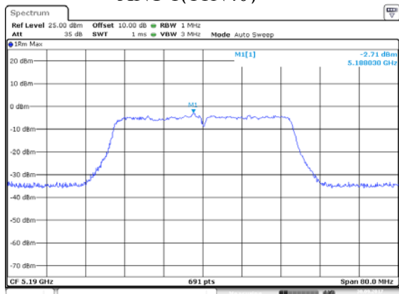
ANT 1(11N40)
