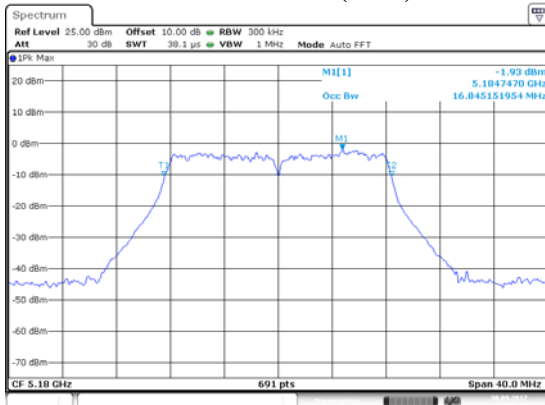
ANT 1(11A)
