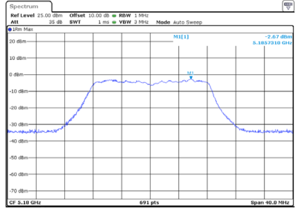
ANT 2(11A)
