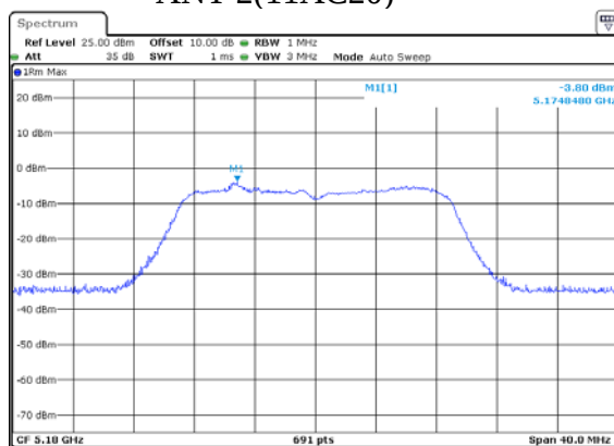
ANT 2(11AC20)
