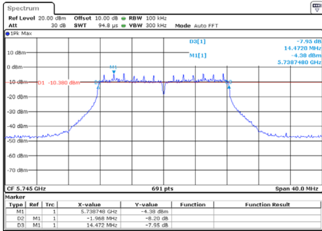
ANT 1(802.11A)
