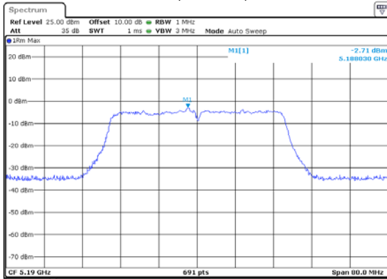
ANT 1(11N40)
