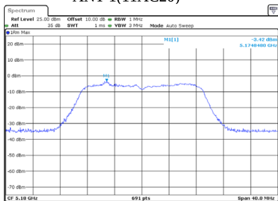
ANT 1(11AC20)
