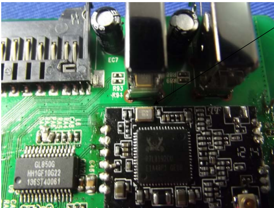
40MHz Crystal
