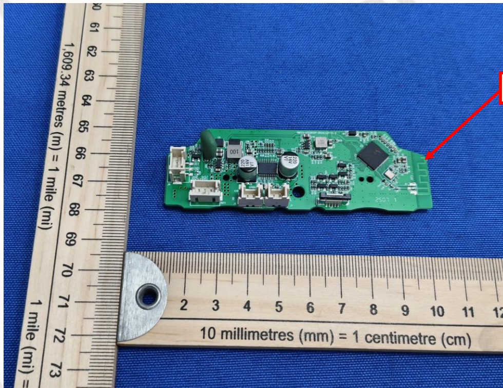
BLE Antenna
