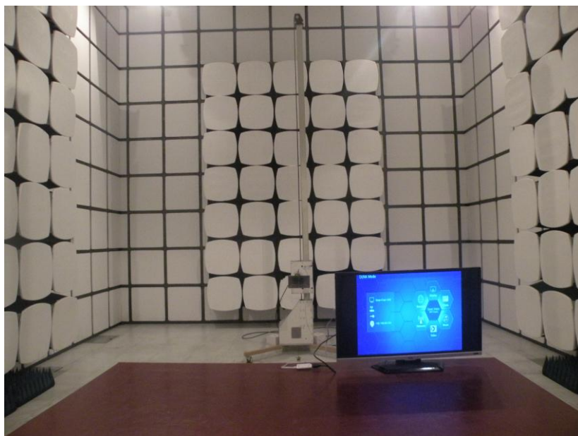
Above 1G
