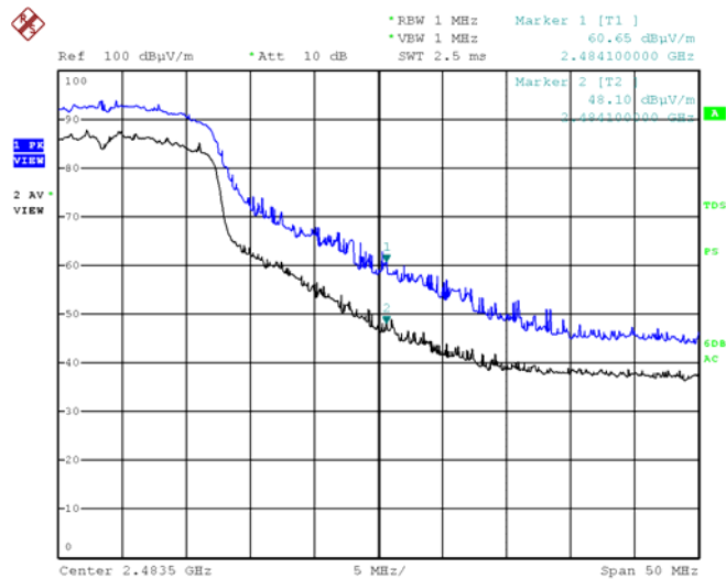
802.11n(ht20) High (Horizontal)
