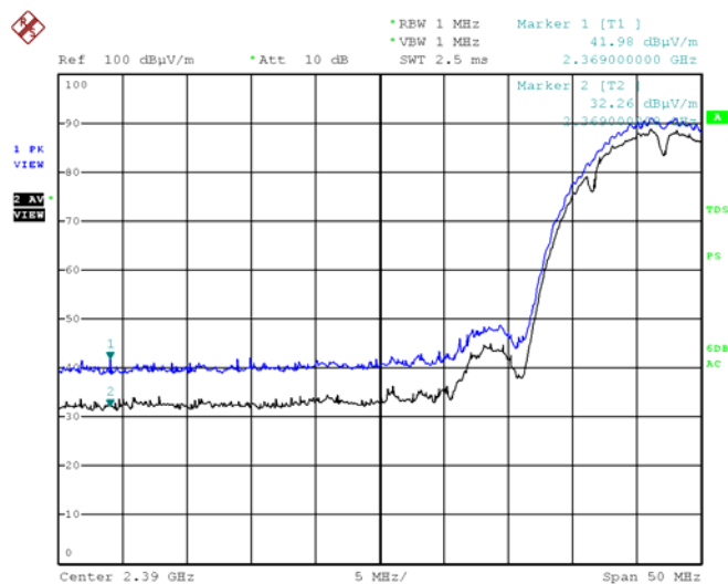
802.11b Low (Vertical)
