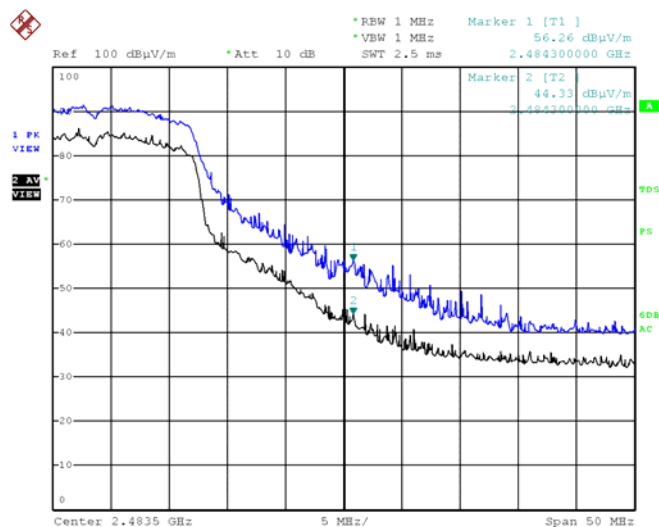
802.11n(ht20) High (Vertical)
