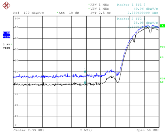
802.11b Low (Horizontal)
