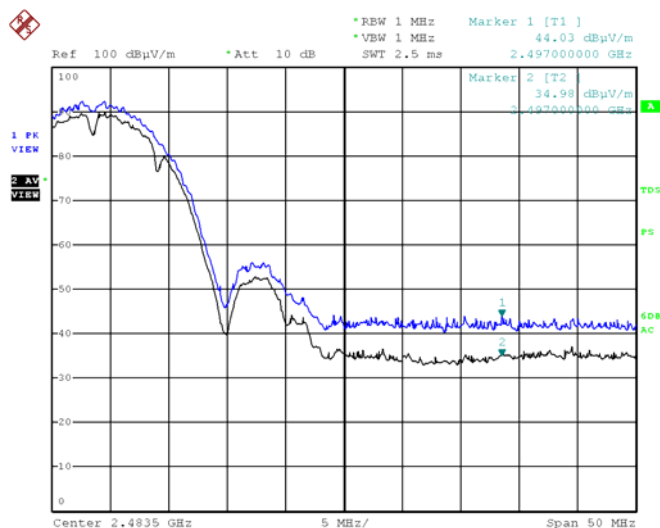
802.11b High (Vertical)
