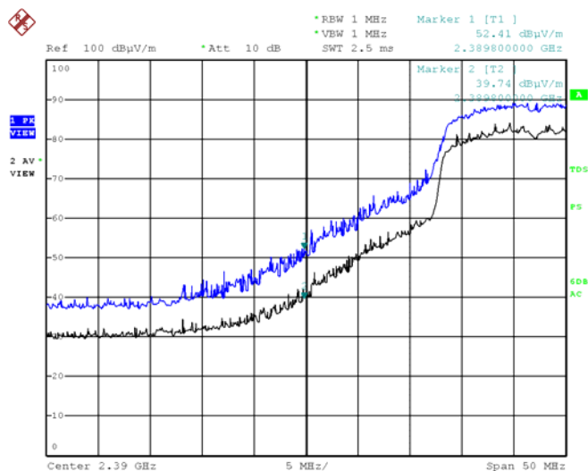
802.11n(ht20) Low (Vertical)
