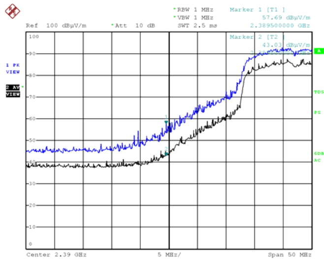
802.11n(ht20) Low (Horizontal)
