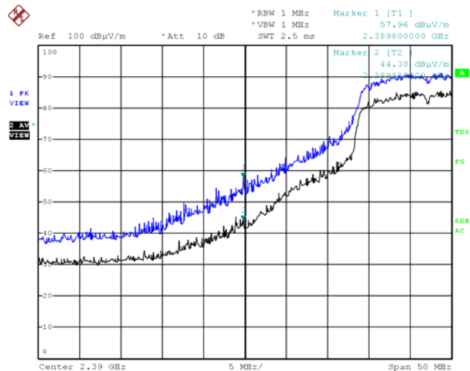
802.11g Low (Vertical)
