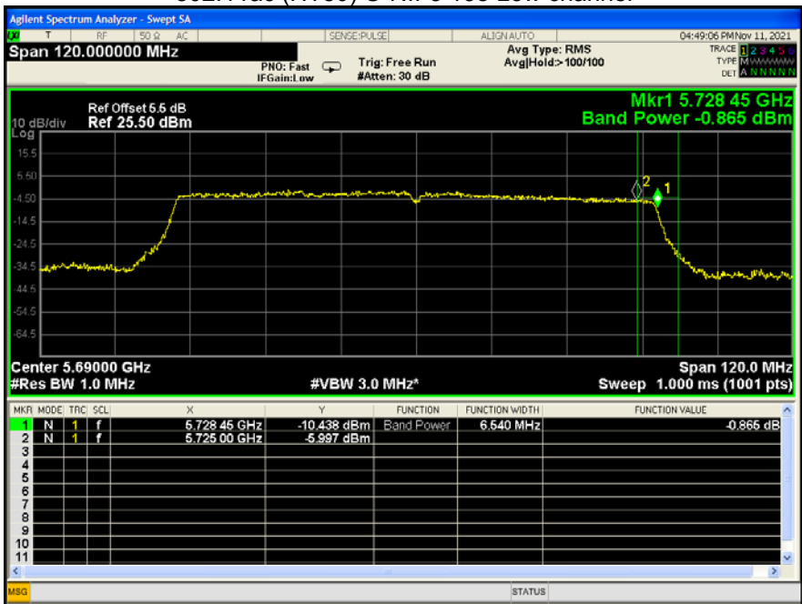
802.11ac (HT80) U-NII-3 138 Low channel
